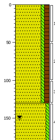
Boring: 4 Datum: 2-10-2020 Boormeester: Ruben van de Bunt
