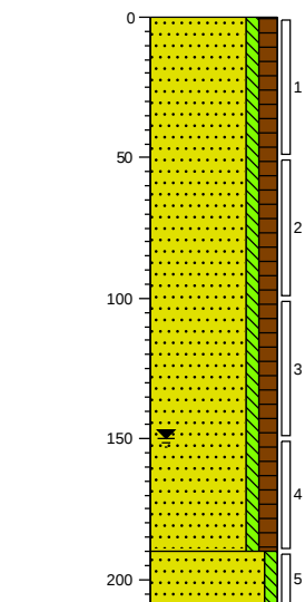
Boring: 3 Datum: 2-10-2020 Boormeester: Ruben van de Bunt
