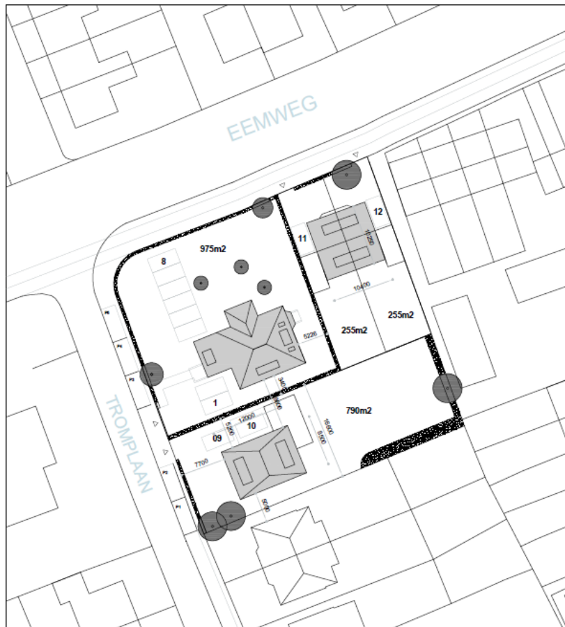
Figuur 1 Bouwkundige tekening van Exit 5 (05-08-2019)
