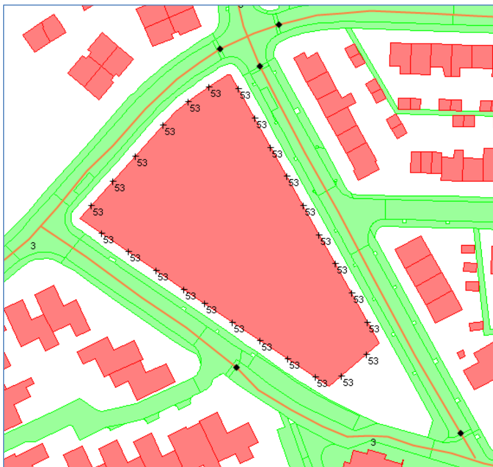
Figuur 4 Hoogst berekende geluidbelasting vanwege de A1 inclusief aftrek conform artikel 110 g Wgh voor het deelgebied 2 John F. Kennedylaan
