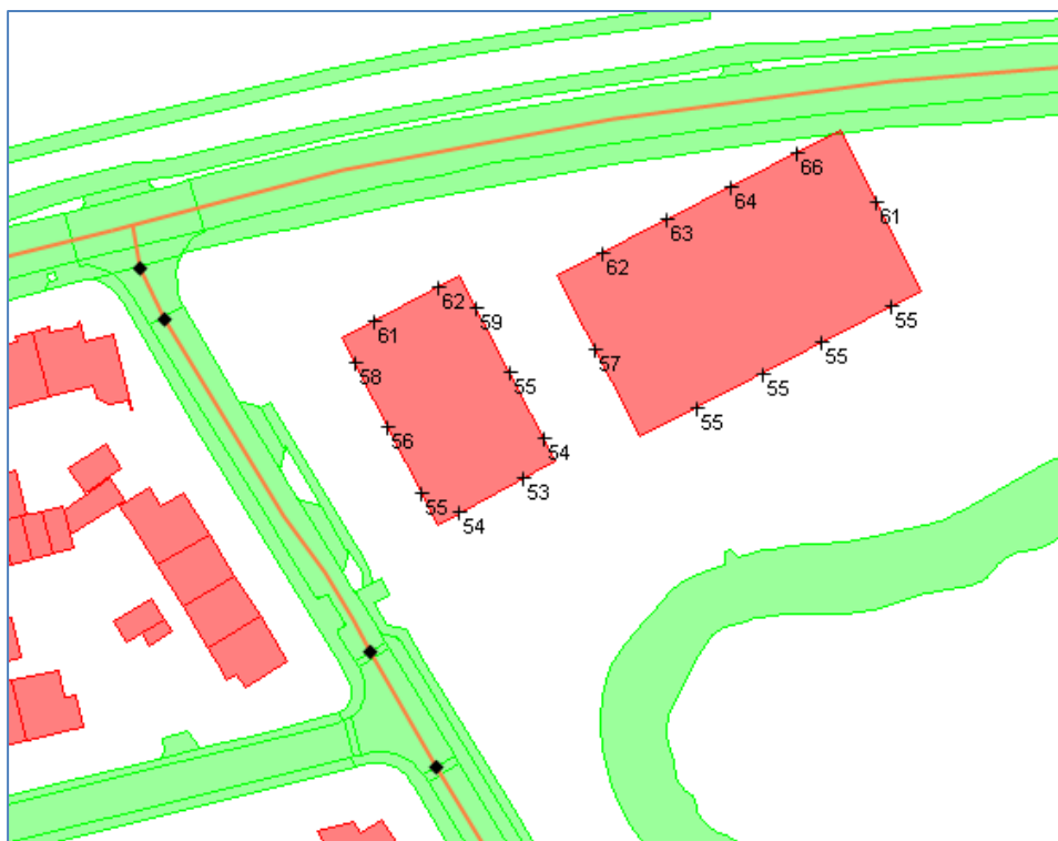
Figuur 6 Hoogst berekende gecumuleerde geluidbelasting (exclusief aftrek artikel 110 g Wgh) op het deelgebied 1 Drakenburgerweg
