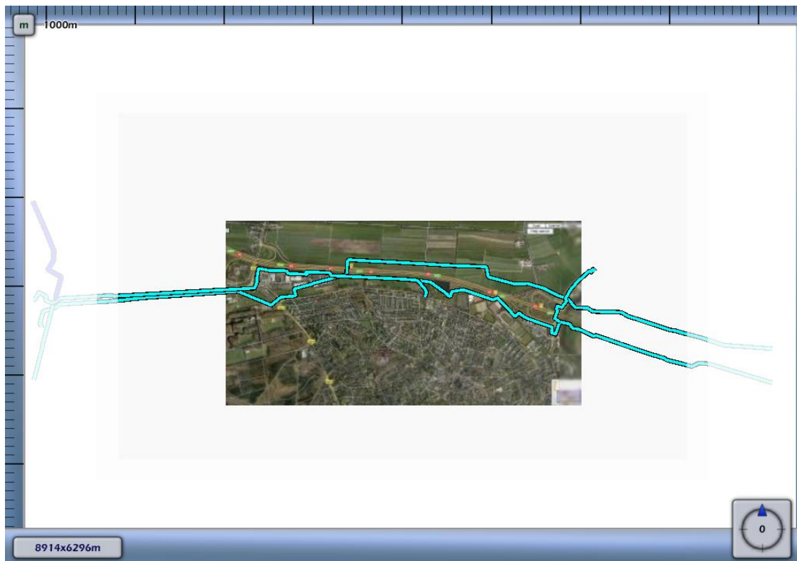
3.7 Figuur 3.7 Plaatsgebonden risico voor W-533-01 van N.V. Nederlandse Gasunie
