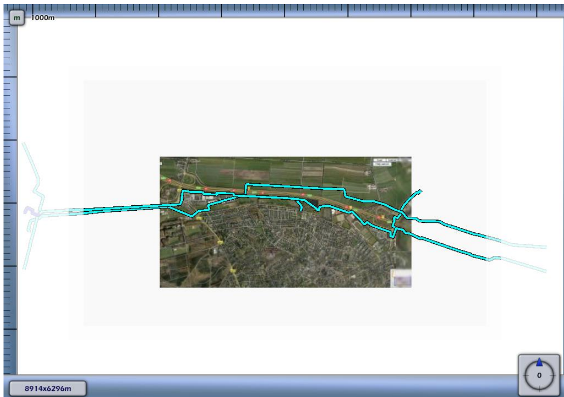
3.3 Figuur 3.3 Plaatsgebonden risico voor W-500-03 van N.V. Nederlandse Gasunie
