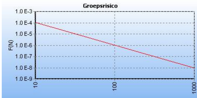
5.7 Figuur 5.7 FN curve voor W-533-01 van N.V. Nederlandse Gasunie voor de kilometer tussen stationing 0.00 en stationing 0.00
