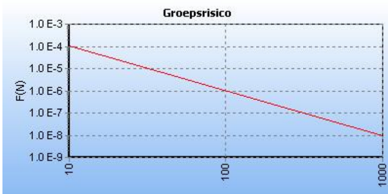
5.5 Figuur 5.5 FN curve voor W-500-21 van N.V. Nederlandse Gasunie voor de kilometer tussen stationing 0.00 en stationing 900.00
