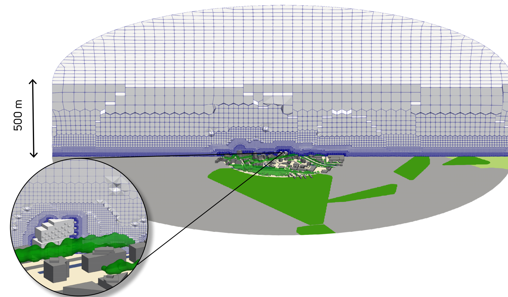
Figuur 3.2: Doorsnede van het rekenrooster Zicht vanuit het zuiden
