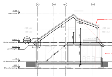
DOORSNEDE D-D
