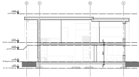
DOORSNEDE A-A
