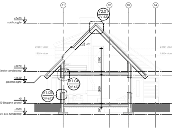
DOORSNEDE B-B
