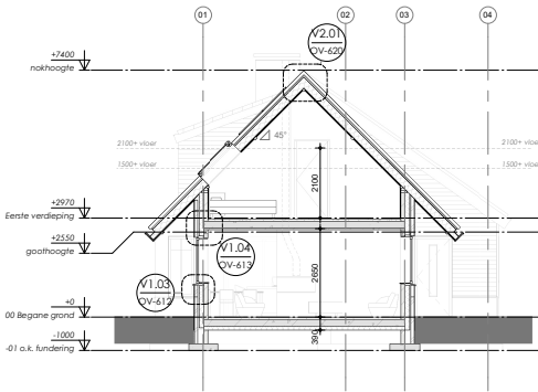
DOORSNEDE B-B
