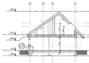
DOORSNEDE C-C
