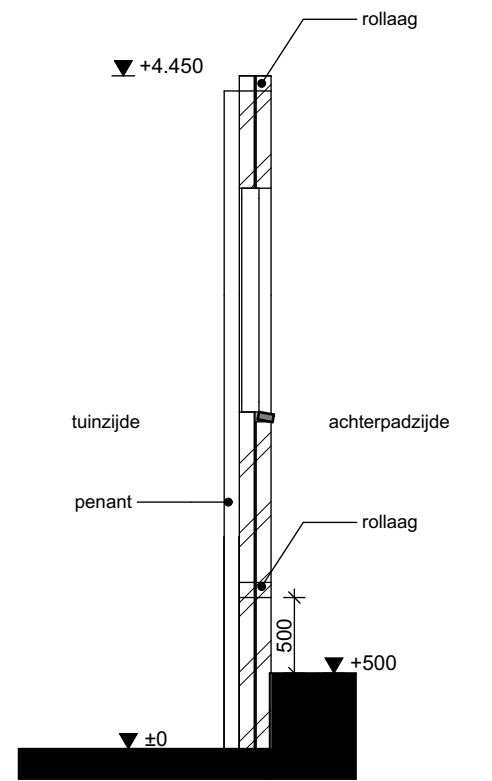
Doorsnede (bestaand)
