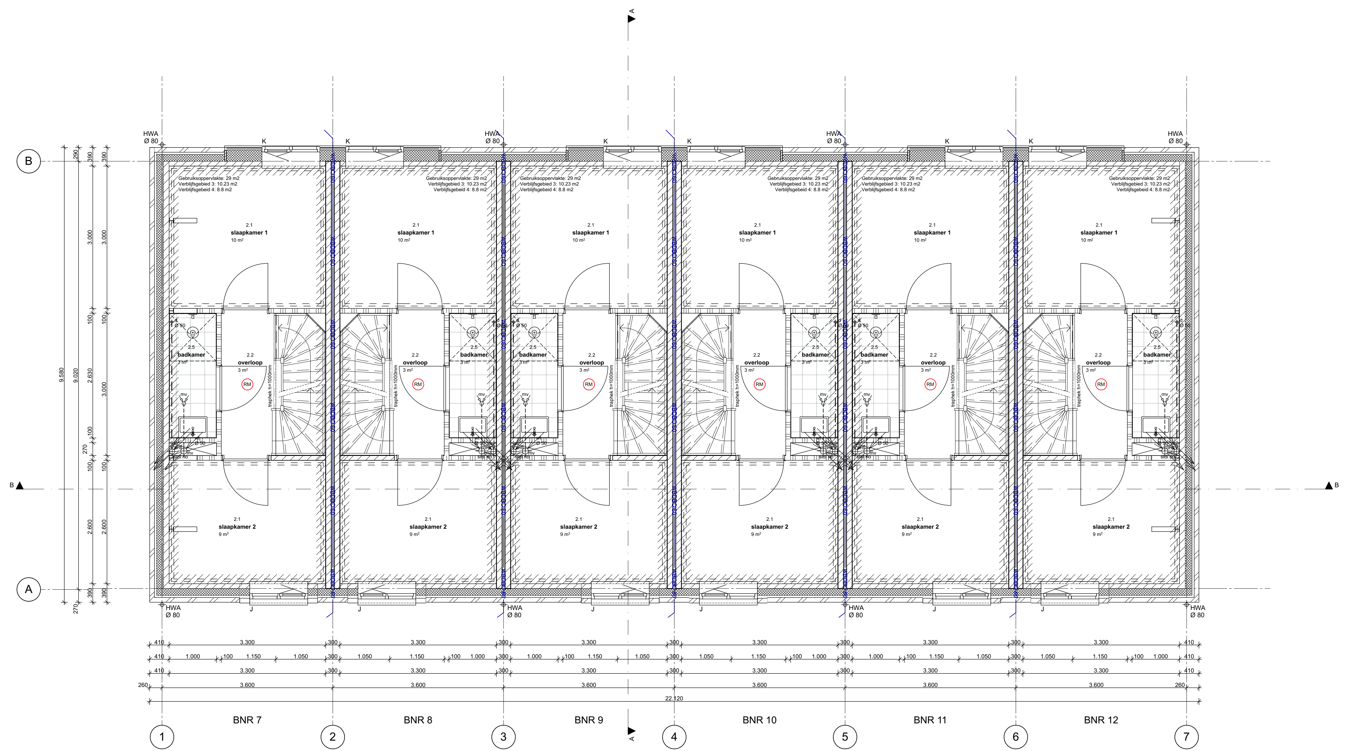
1e verdieping
