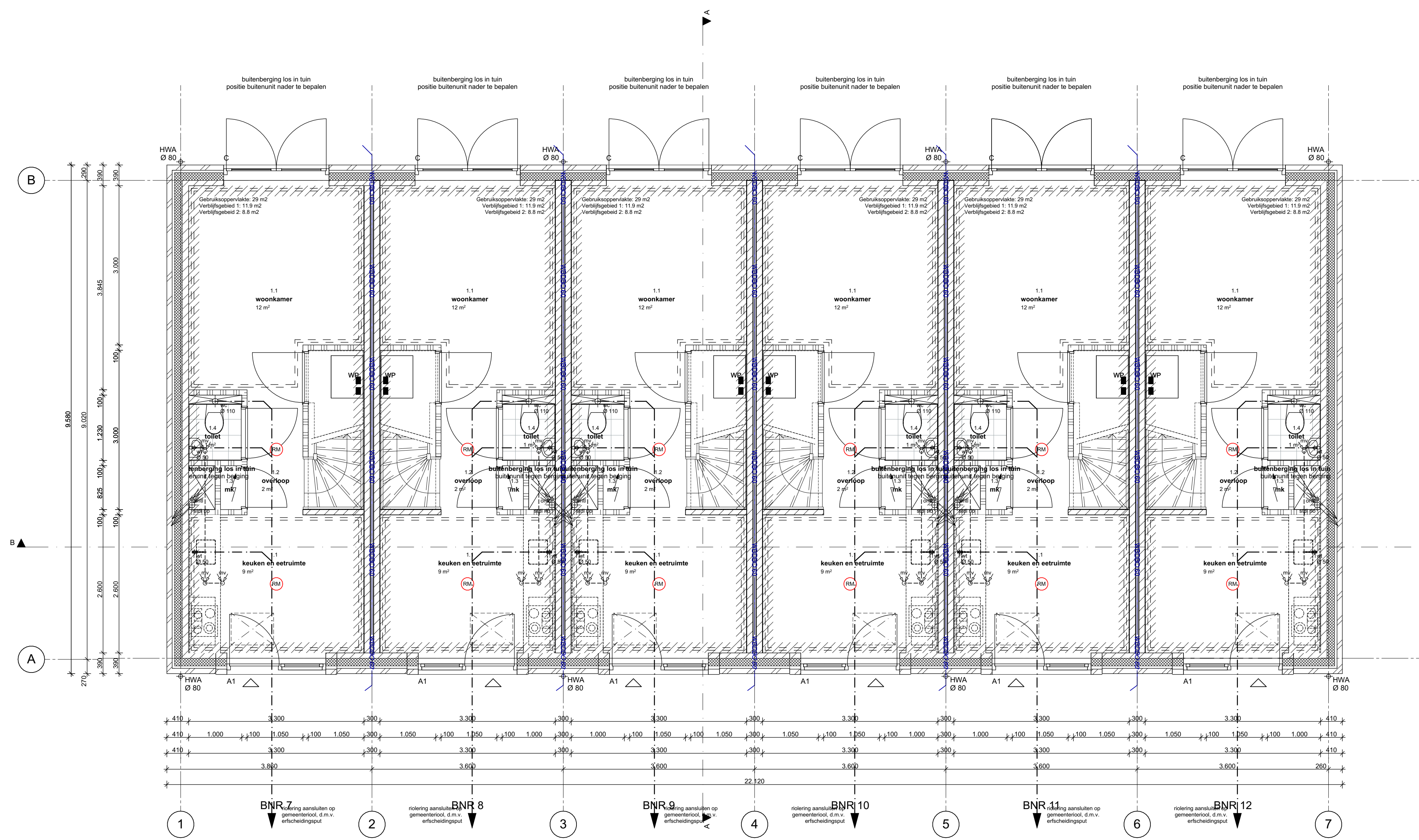
begane grond
