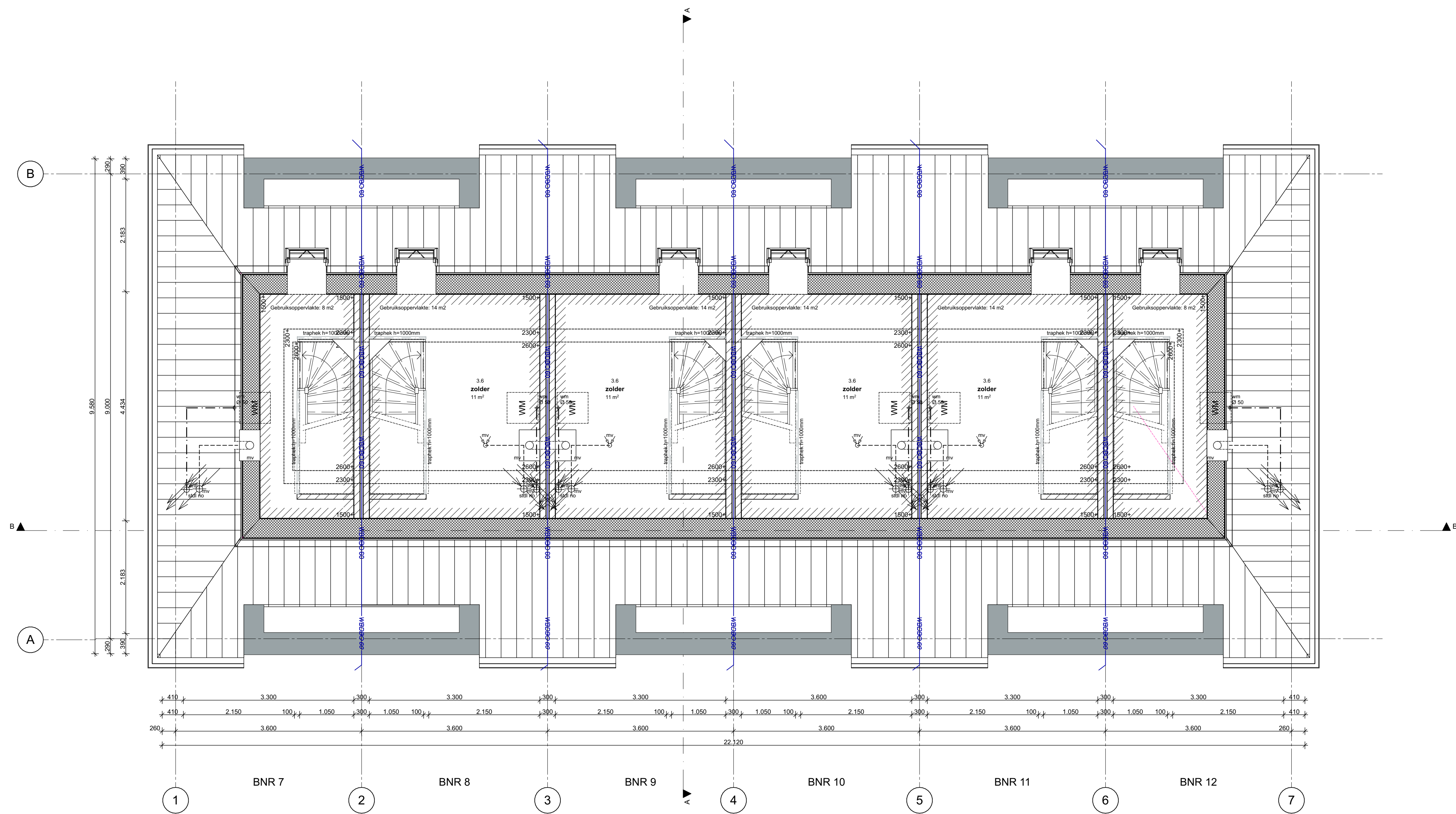
2e verdieping
