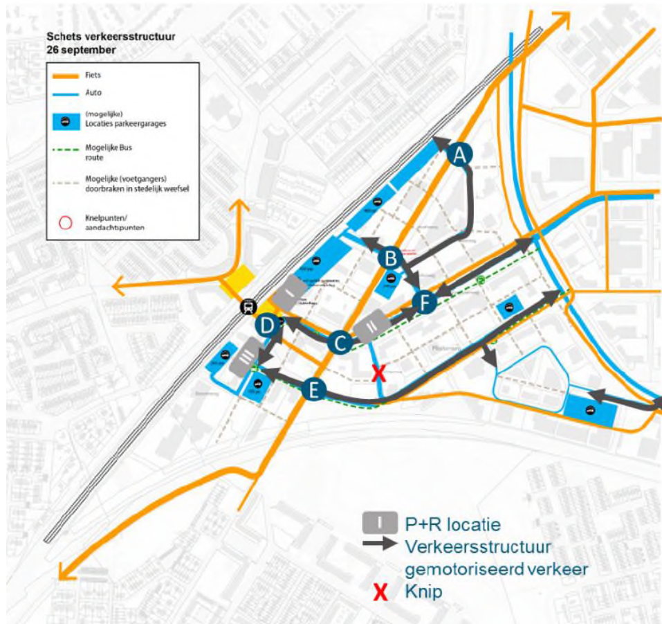
Figuur 0.5: Schets verkeerstructuur variant 3
