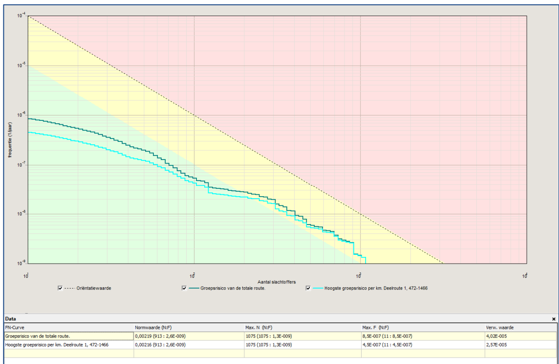
Afbeelding 5 fN-curve berekend groepsrisico, toekomstige situatie
