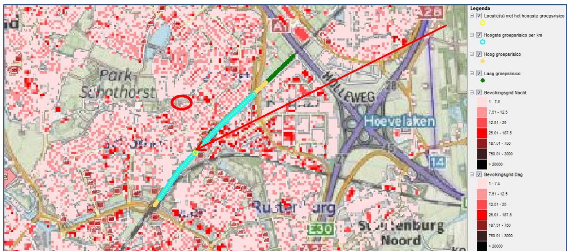
Afbeelding 4 Locatie met hoogte GR spoorweg, huidige situatie
