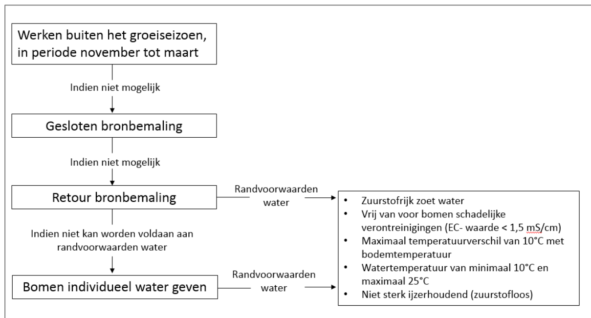
figuur 6: stappenplan bronbemaling
