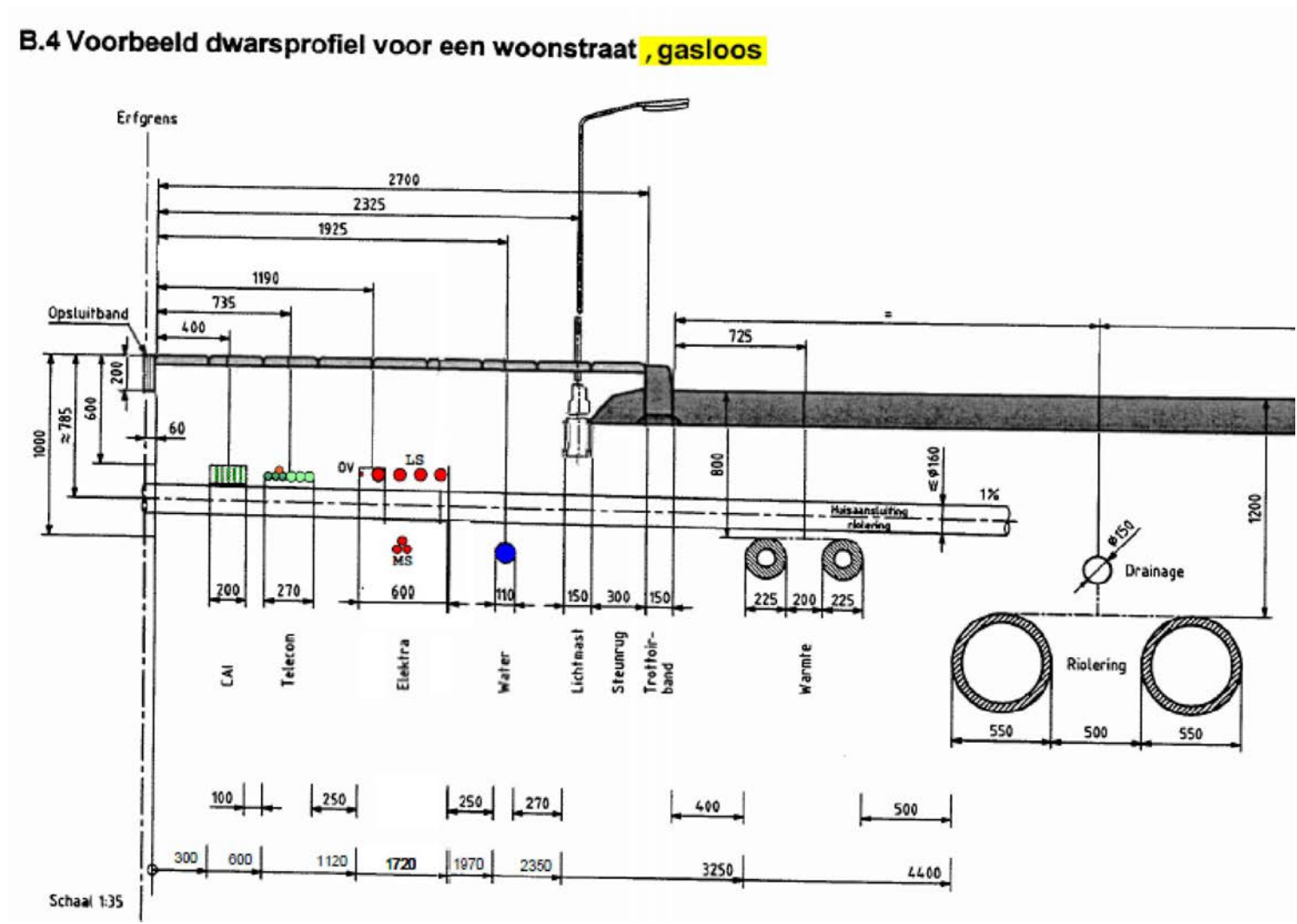
Voorbeeld dwarsprofiel (Let op nog afstemmen met de combi)
