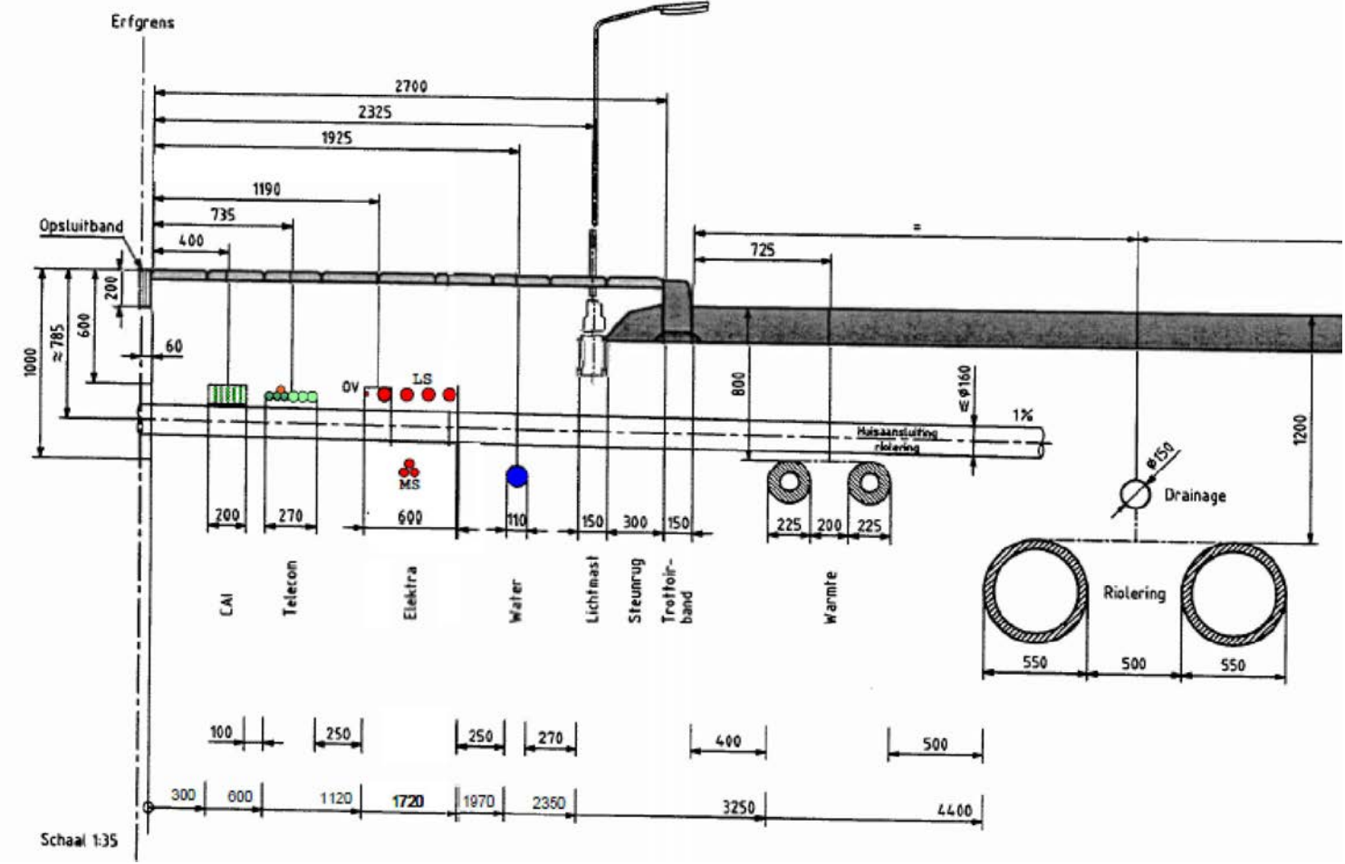
B.4 Voorbeeld dwarsprofiel voor een woonstraat, gasloos
