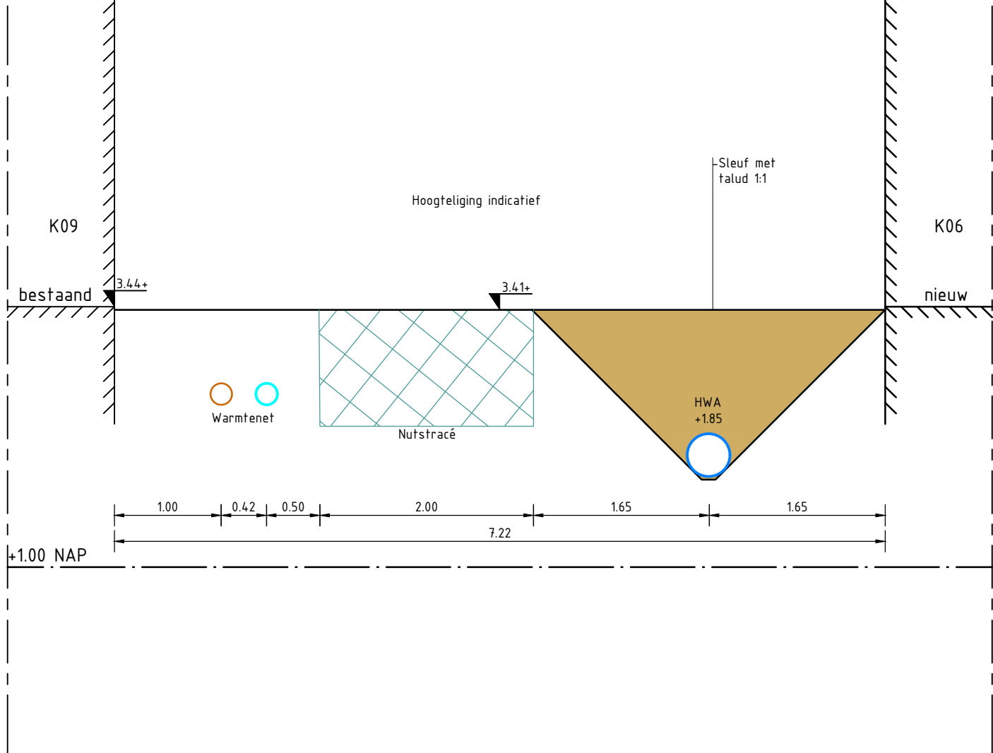
Doorsnede D-D
