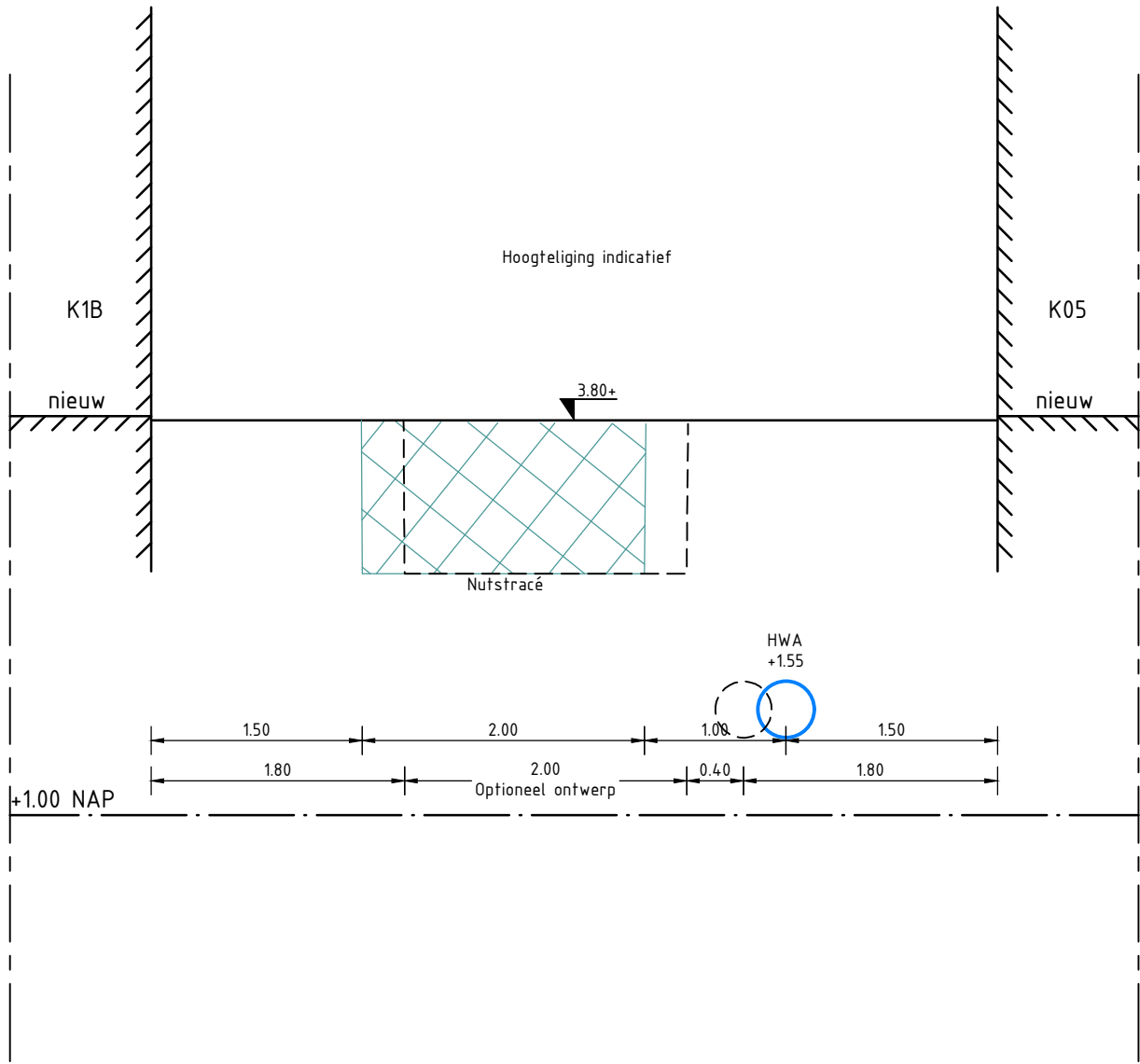
Doorsnede B-B
