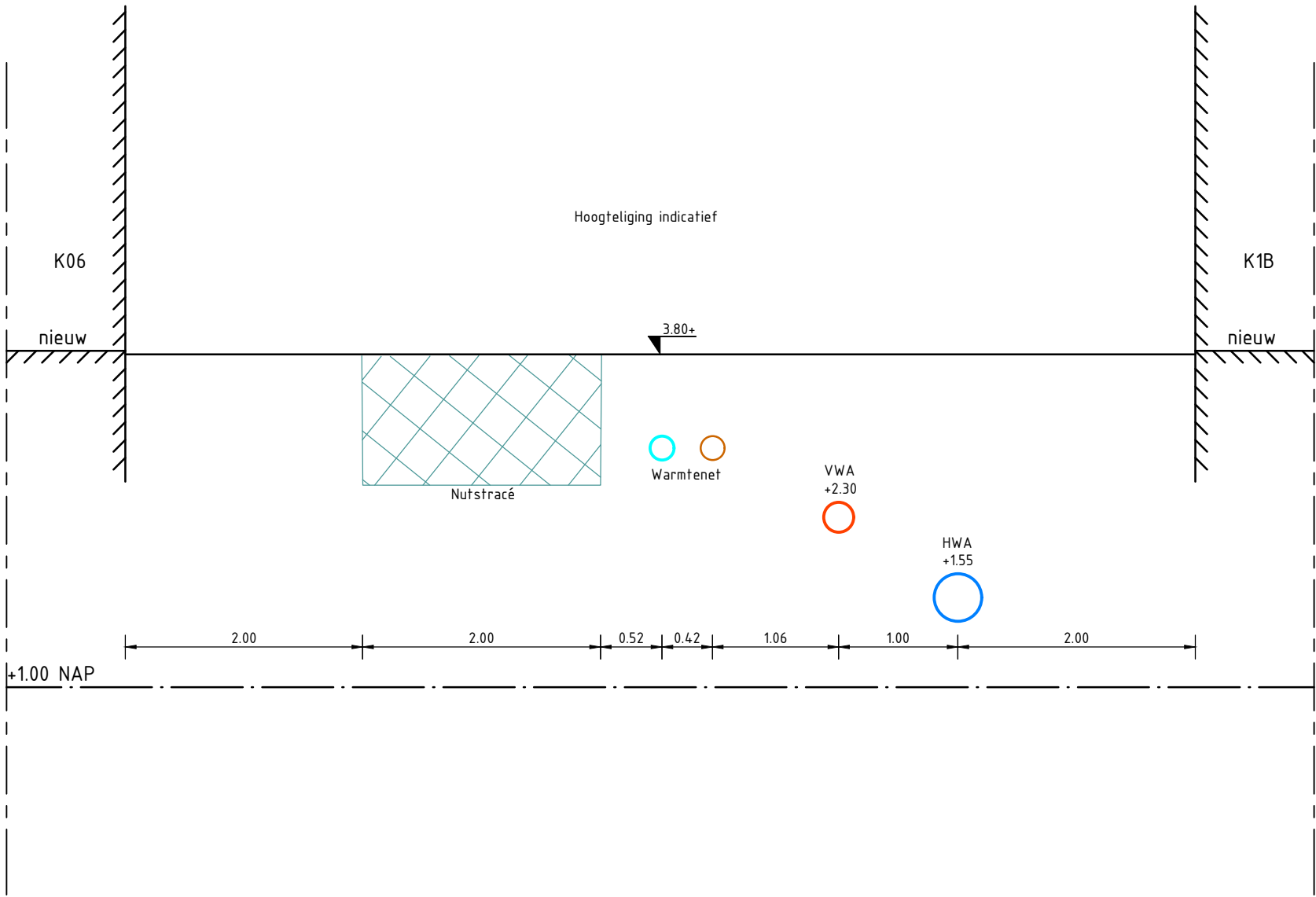
Doorsnede A-A (voorbeeld van gewenste situatie op basis van principeprofiel nutstracé)
