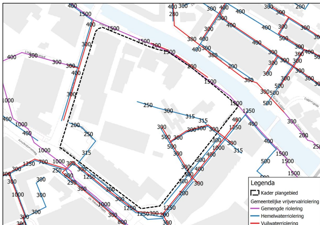
Figuur 2-4: Gemeentelijke riolerings binnen en in omgeving plangebied (bron: GWSW)
