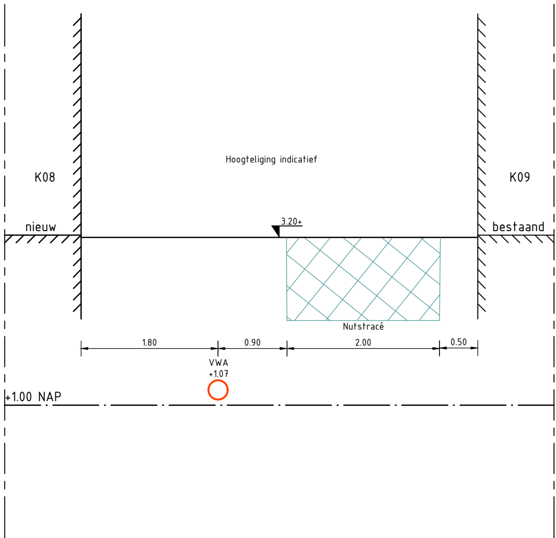
Doorsnede C-C
