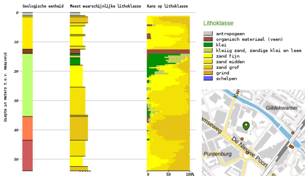
Figuur 2-3: Geologische eenheid en lithoklasse op basis van profiel DINOlaket, model GeoTOP v1.4.1 (2022)
