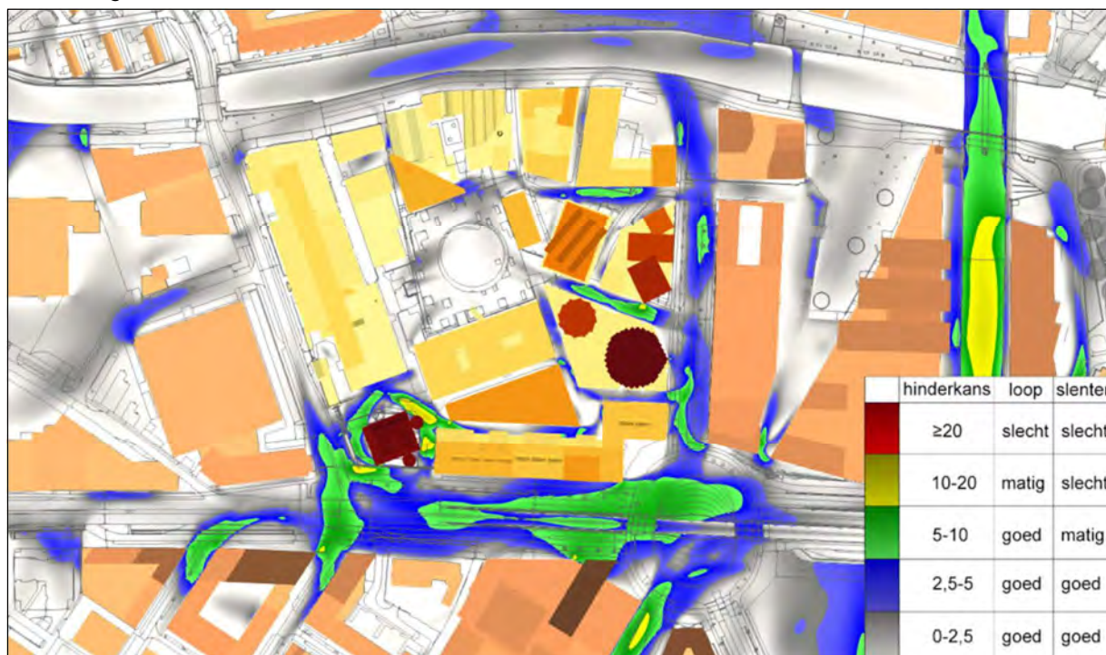
Afbeelding 22: Verwachte windklimaat NEN 8100
