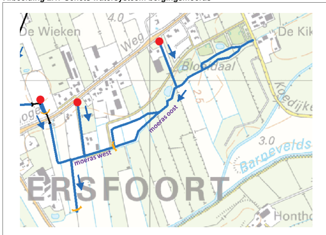
Afbeelding 2.1. Schets watersysteem bergingsmoeras
