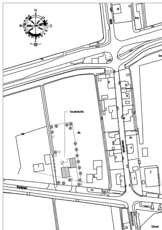
NIEUWE SITUATIE
