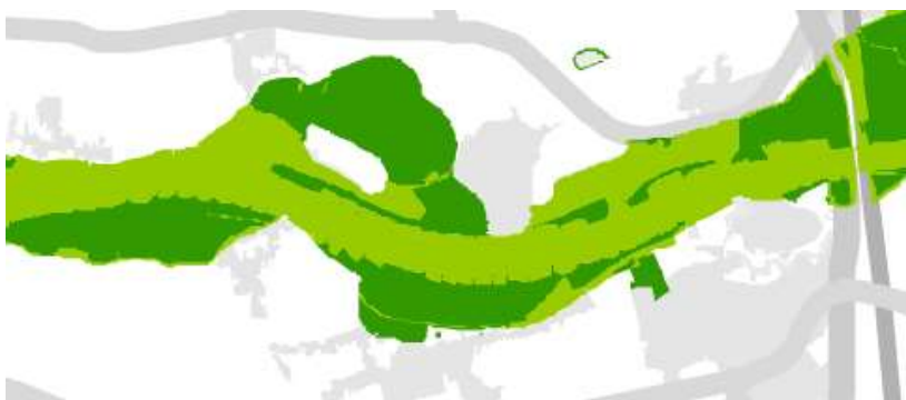
Figuur 4.3 Omgevingsverordening, kaartbeeld Natuur. Donkergroen: Gelders Natuurnetwerk; lichtgroen: Groene ontwikkelingszone.
