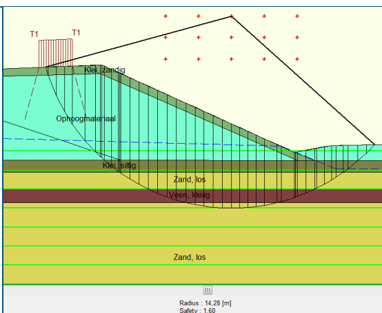
Glijcirkel dwp 4, Bishop bij een Minimum Circle Depth 6,5 m (veiligheidsfactor 1,60)
