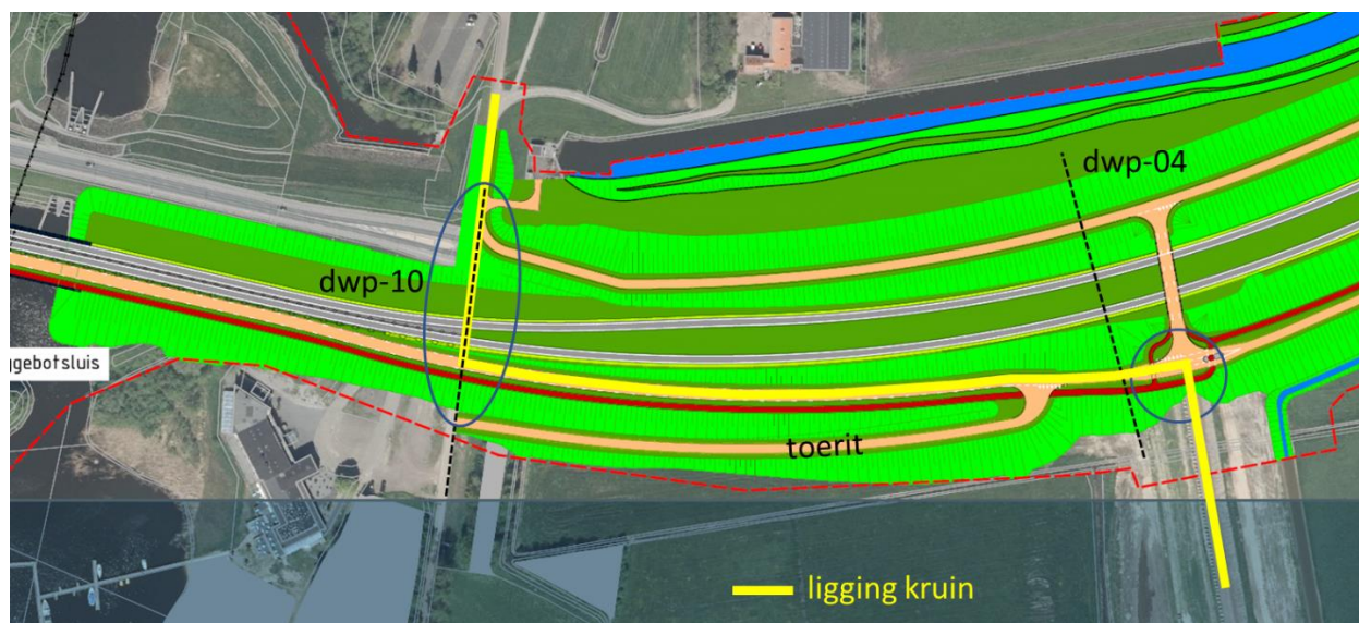
Figuur 2-1: Ligging van de kering in de dijkvakken N11 en N11A, met daarin de ligging van de dwarsprofielen in de berekening.
