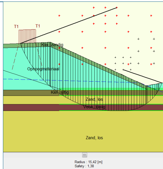
Glijcirkel dwp 4, Uplift-Van bij een Minimum Circle Depth 6,5 m (veiligheidsfactor 1,38)
