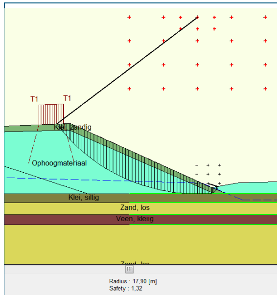
Glijcirkel dwp 4, Uplift-Van (veiligheidsfactor 1,32)
