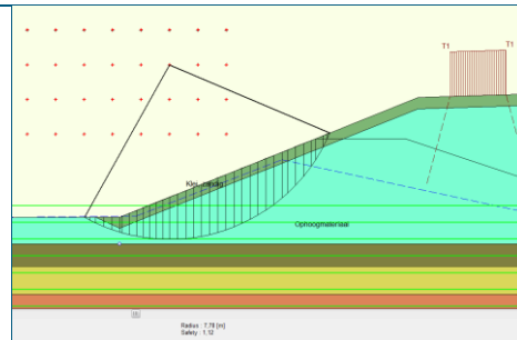
Glijcirkel dwp-10, Bishop bij een talud 1:2,5 (veiligheidsfactor 1,13)
