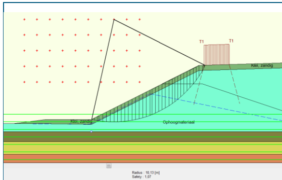
Glijcirkel dwp-10, Bishop bij een talud 1:2 (veiligheidsfactor 1,07)
