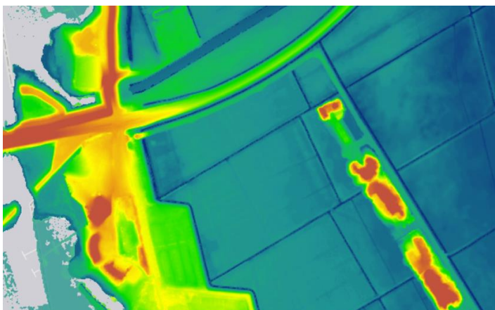
Figuur 3-2: Hoogtegegevens dijkvak N11 (bron: AHN)
