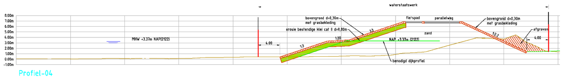
Figuur 2-3: Dijkontwerp ter plaatse van dwp-04
