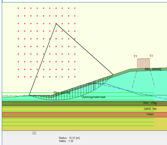
Glijcirkel dwp-10, Bishop bij een talud 1:3 (veiligheidsfactor 1,36)
