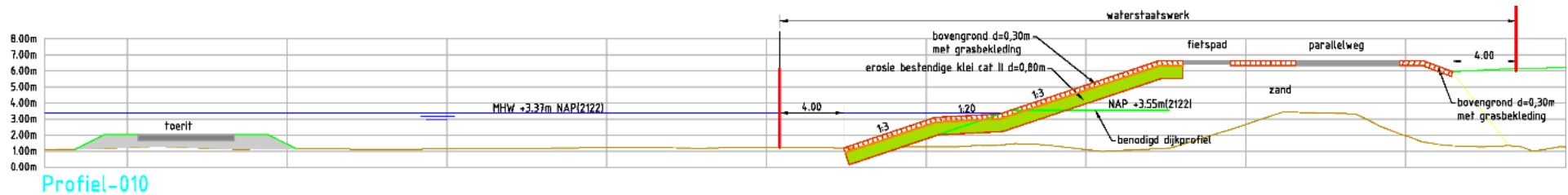
Figuur 2-2: Dijkontwerp ter plaatse van dwp-010
