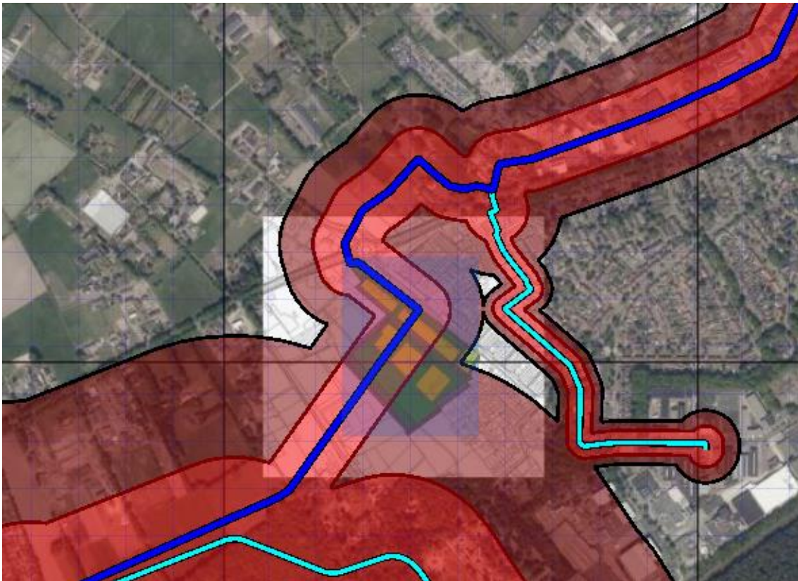
Afbeelding 2 Invloedsgebieden buisleidingen (bron: CAROLA)
