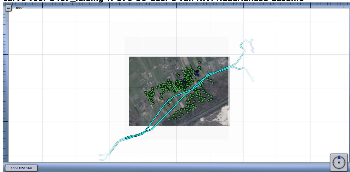
Figuur 4.3 Kilometer leiding behorende bij de maximale overschrijding van de FN-curve voor 8417_leiding-N-570-30-deel-1 van N.V. Nederlandse Gasunie
