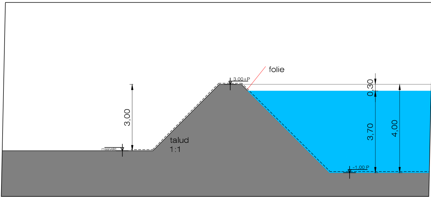
Principeddoorsnede A-A indicatief
