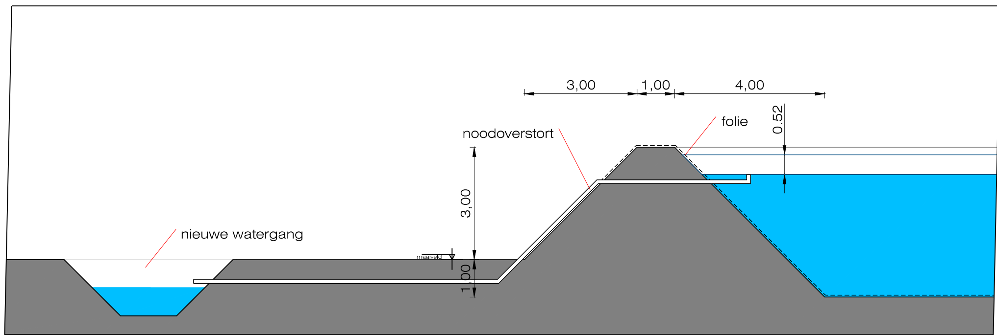
Principeddoorsnede C-C indicatief
