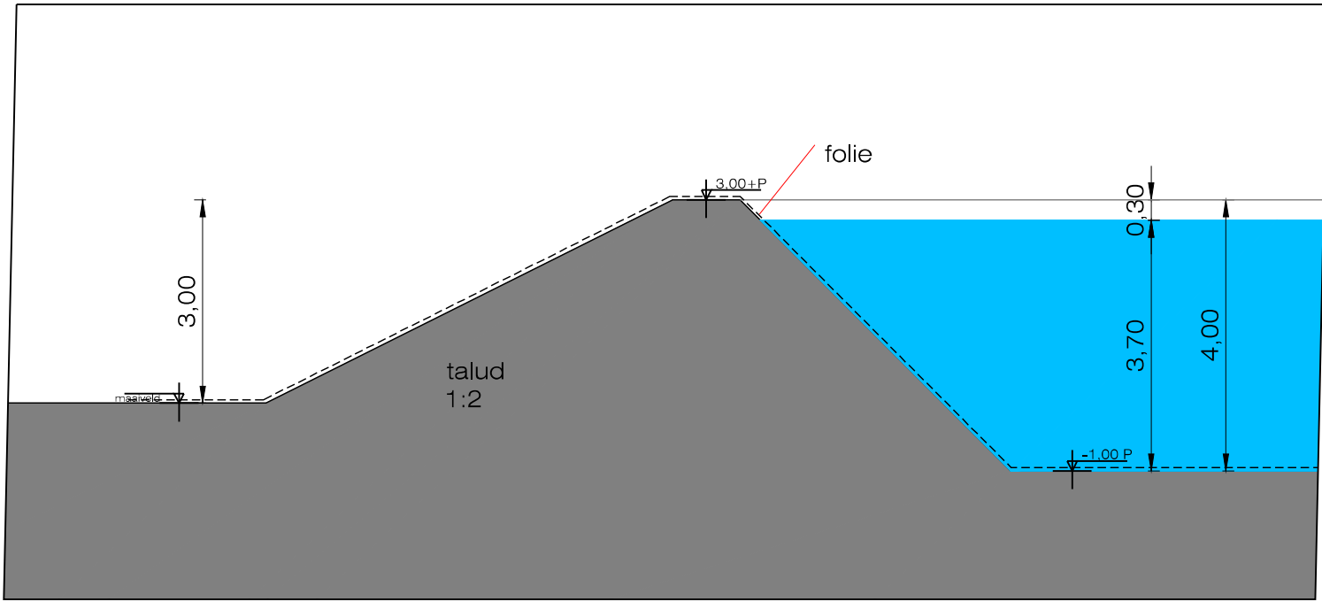
Principeddoorsnede B-B indicatief
