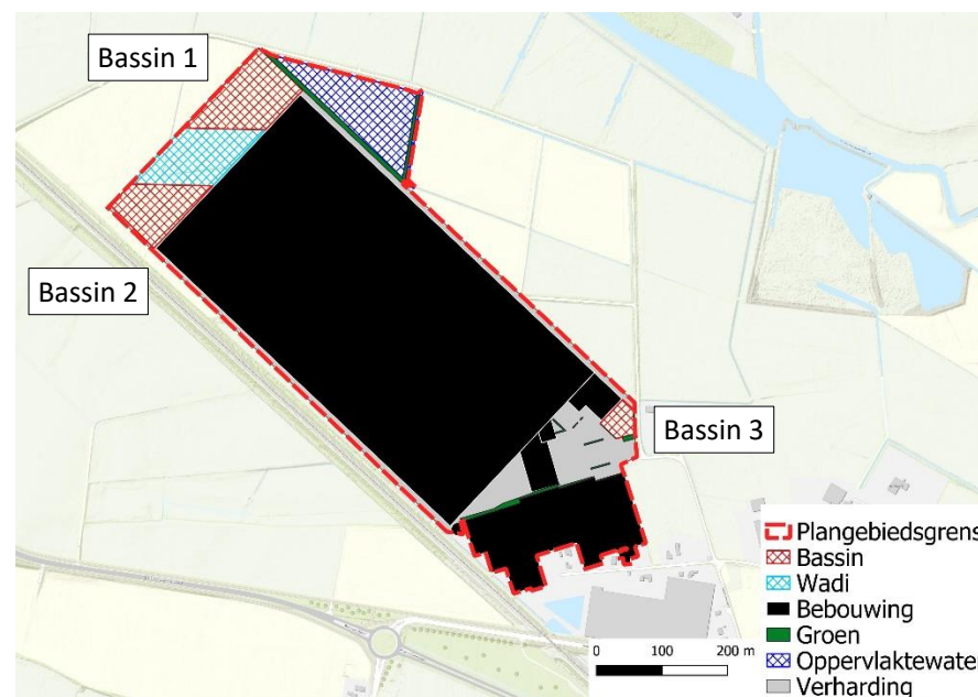
Figuur 4-1: Ruimtelijke weergave waterbergende voorzieningen
