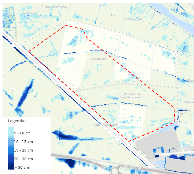
Figuur 2-5: Waterdiepte bij hevige bui, 70mm/2 uur (Klimaateffectatlas, 2018)
