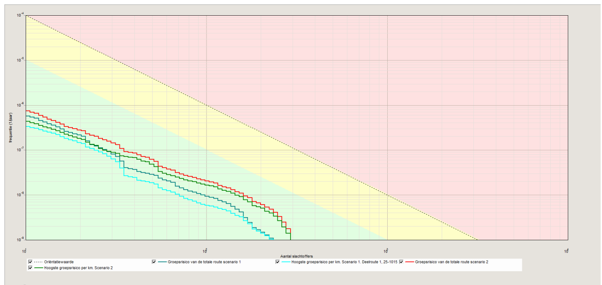
Figuur 4.1 Groepsrisico voor de huidige situatie (scenario 1) en nieuwe situatie voor het plangebied 'de Bem' (scenario 2).
