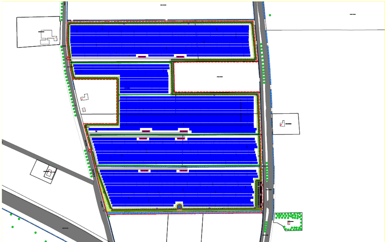
Figuur 4. Huidig inrichtingsplan voor zonnepark Zevenaar (bron: KS NL23). De ruimtelijke invulling met zonnepaneelstellingen is met blauw aangegeven.
