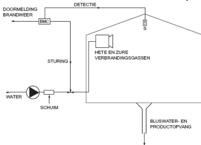
Figuur B1.1 Schematische weergave werkwijze van een Inside-air brandbestrijdingssysteem
