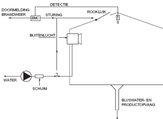
Figuur B1.2 Schematische weergave van de werkwijze van een Outside air brandbestrijdingssysteem
