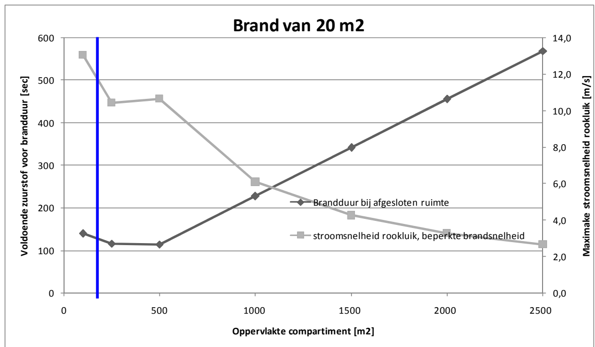
Figuur B3.1. BerekenedBrandduur en stroomsnelheid als functie van de compartiment omvang
