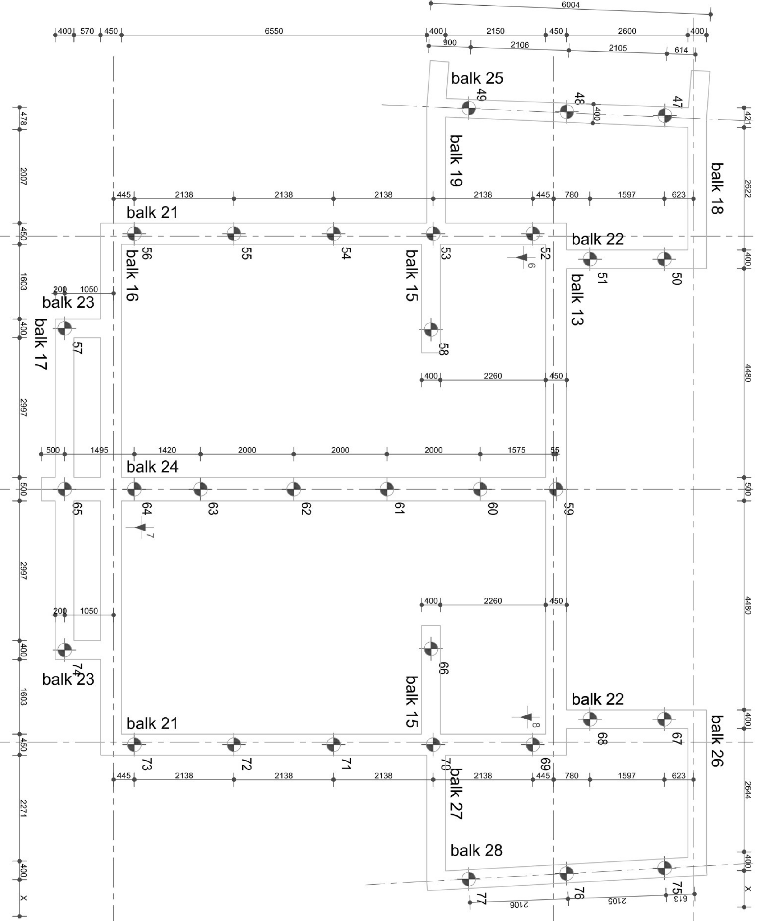
Fundering Nr. 4
