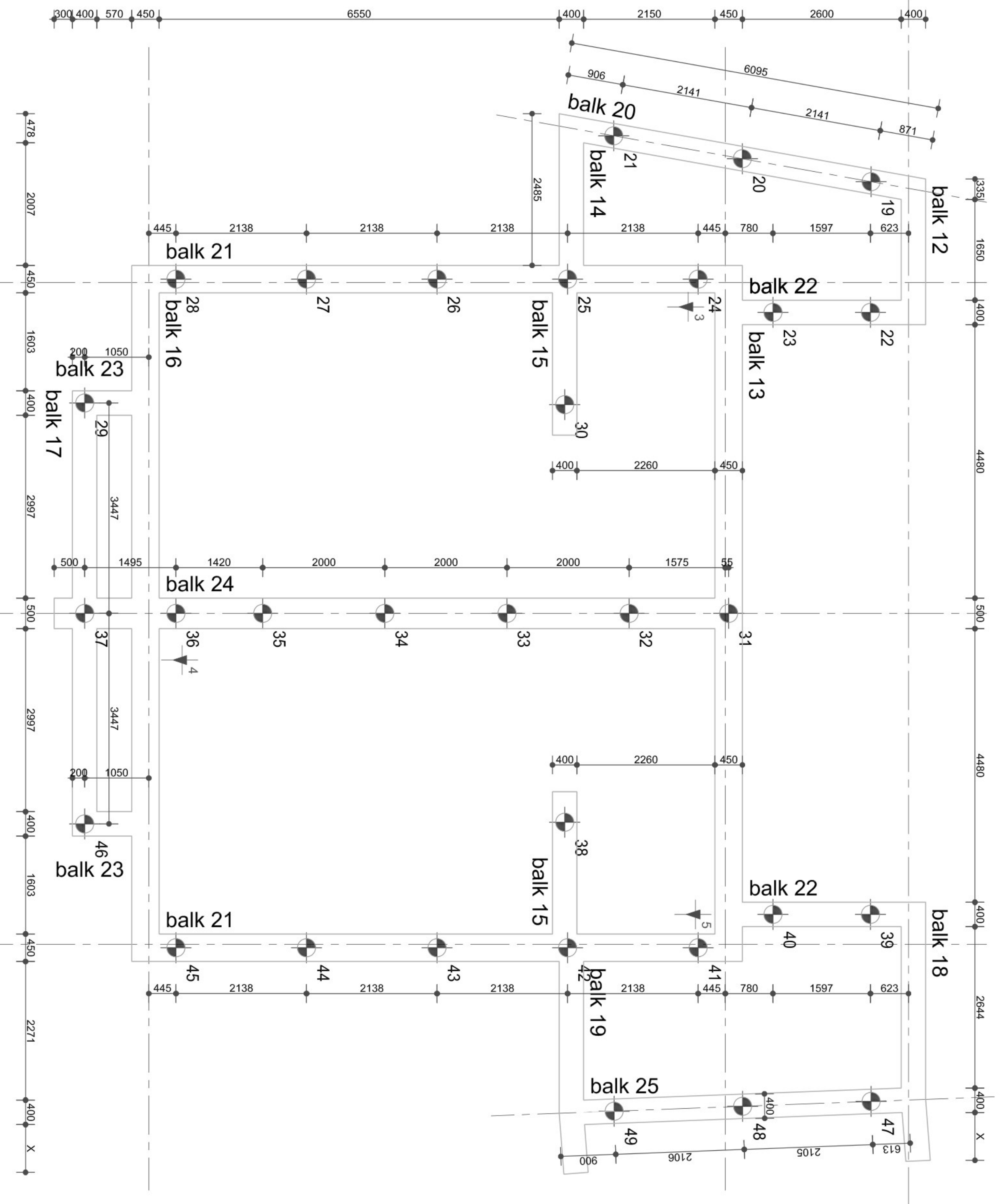
Fundering Nr. 2
