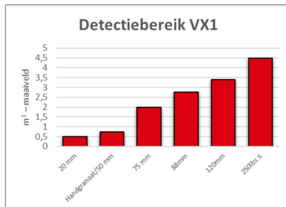
Figuur 7. Passieve realtime oppervlakedetectie met een Vallon VX1 Magnetometer en een staafdiagram waarop het maximale detectiebereik (m 1 – maaiveld) per kaliber.
