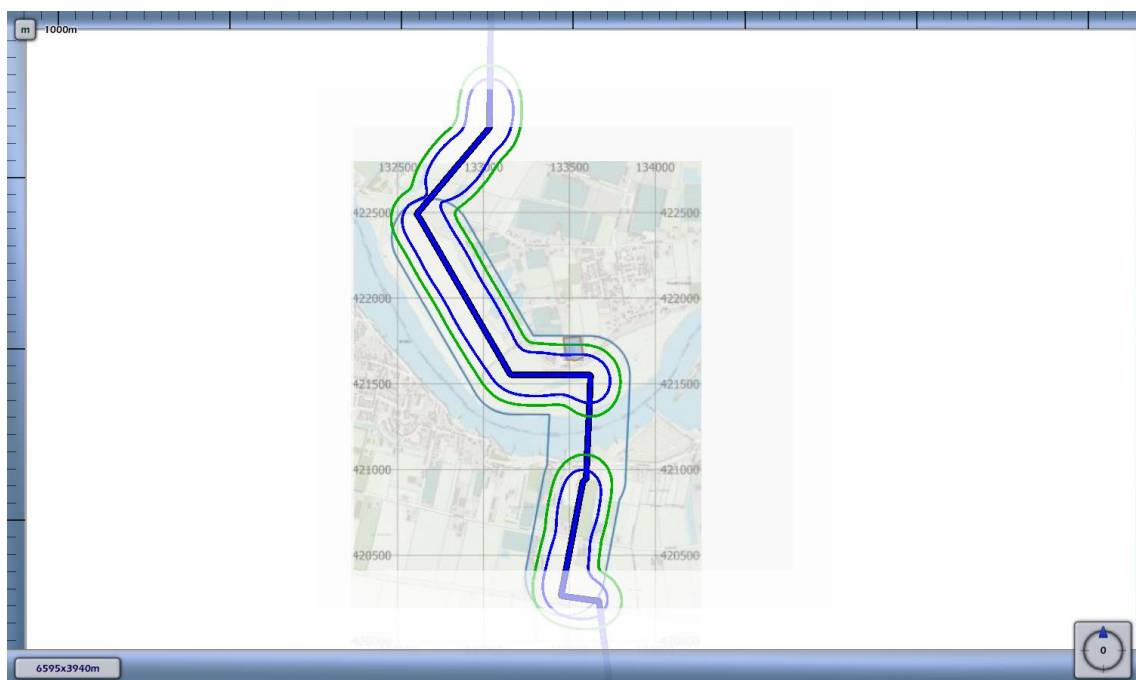
3.1 Figuur 3.1 Plaatsgebonden risico voor 5780_leiding-A-618-deel-1 van N.V. Nederlandse Gasunie
