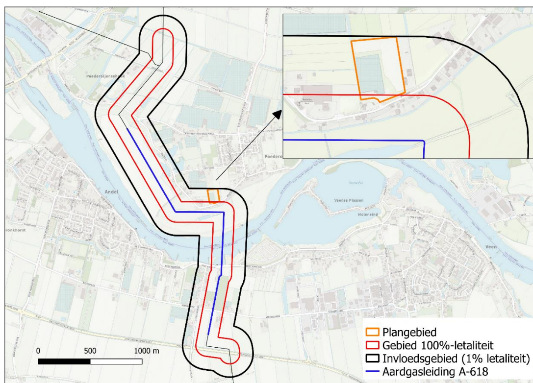
Figuur 2. Aardgasleiding A-618 en het invloedsgebied
