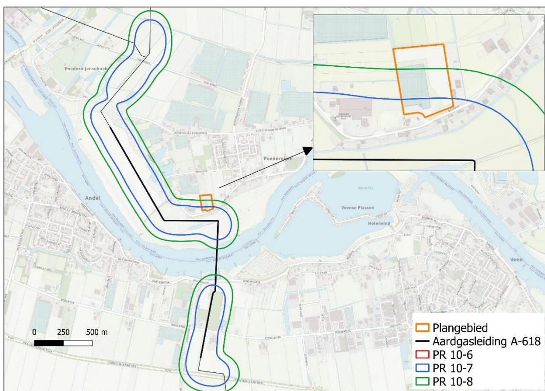
Figuur 3. PR-contouren aardgasleiding A-618
