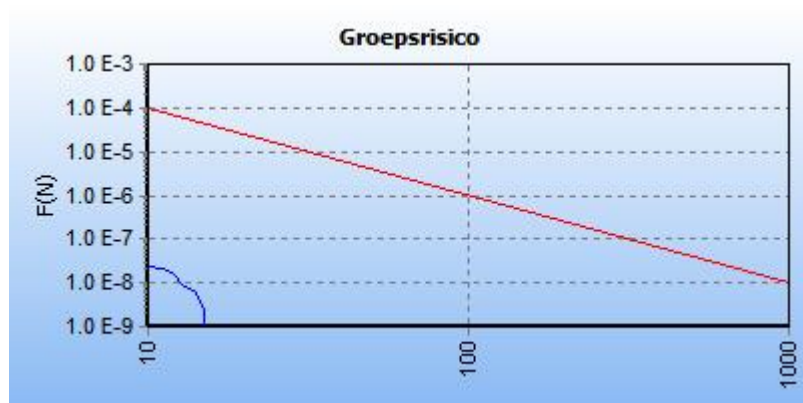
Figuur 4. Groepsrisico A-618 huidige situatie
