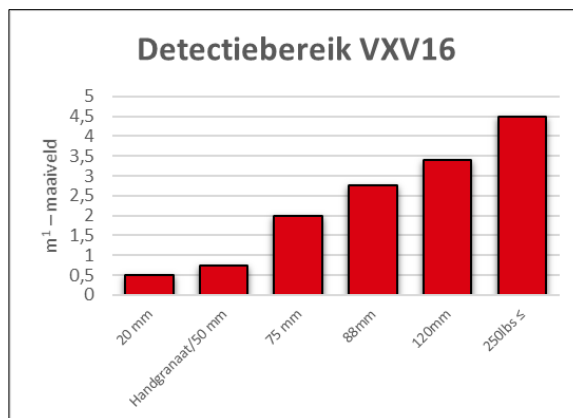
Figuur 3. Passieve non realtime oppervlakedetectie met het Vallon Multisondesysteem VXV16 en een staafdiagram waarop het maximale detectiebereik (m 1 – maaiveld) per kaliber is weergegeven.
