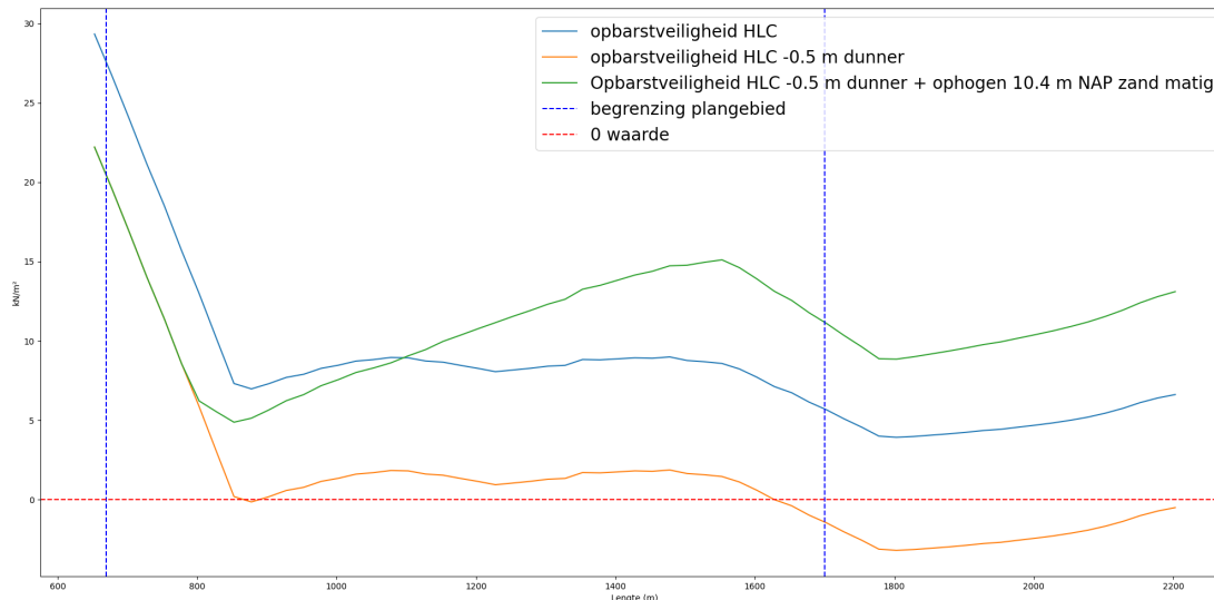
Figuur 6.9 Opbarstrisico verschil tussen gronddruk en opwaarstdruk 1 e watervoerende pakket voor 3 verschillende scenario's
