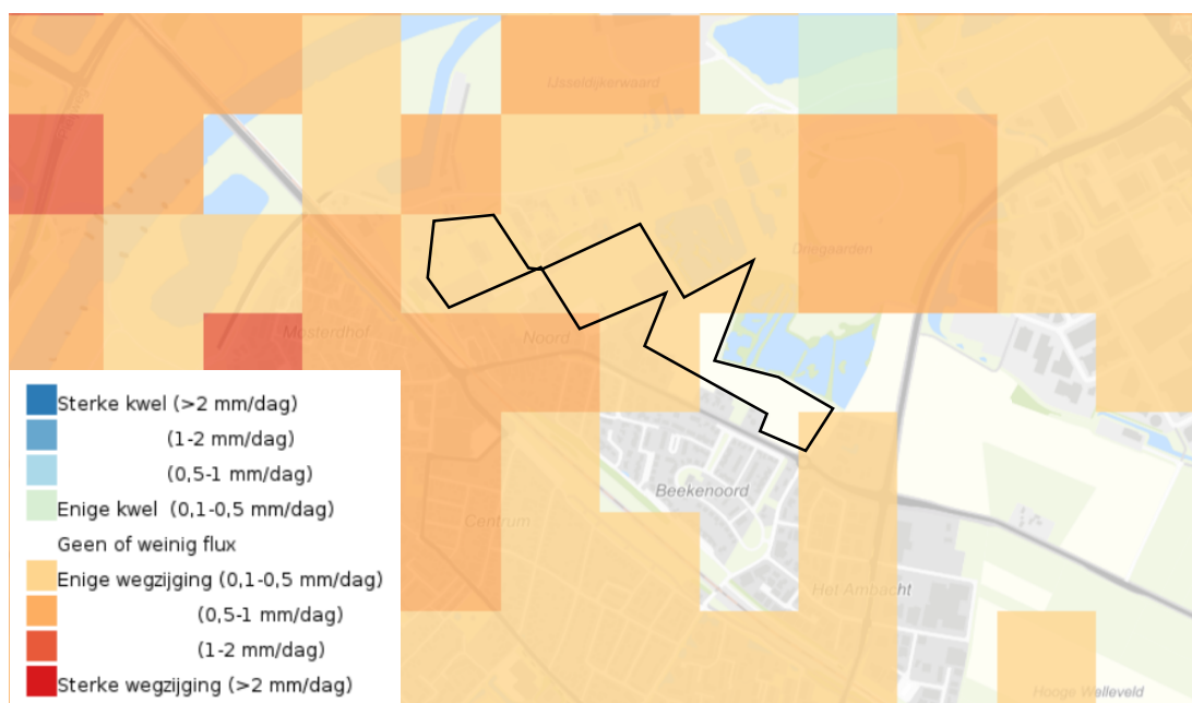
Figuur 2.7 Situatie kwel/wegzijging (bron: Klimaateffectatlas; Deltares Nationaal Water Model 2016)
