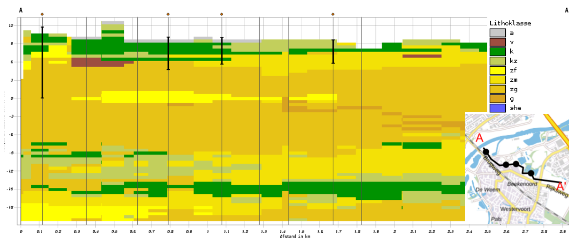
Figuur 2.2 Regionale bodemopbouw (bron: DINOloket GeoTOP)
