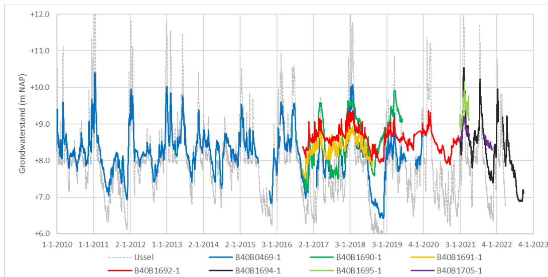
Figuur 2.6 Meetreeks peilbuizen en IJssel (meetpunt RWS Westervoort)
