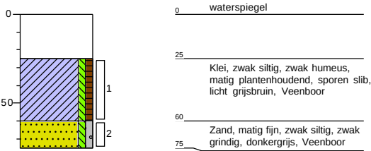
Boring: D10
