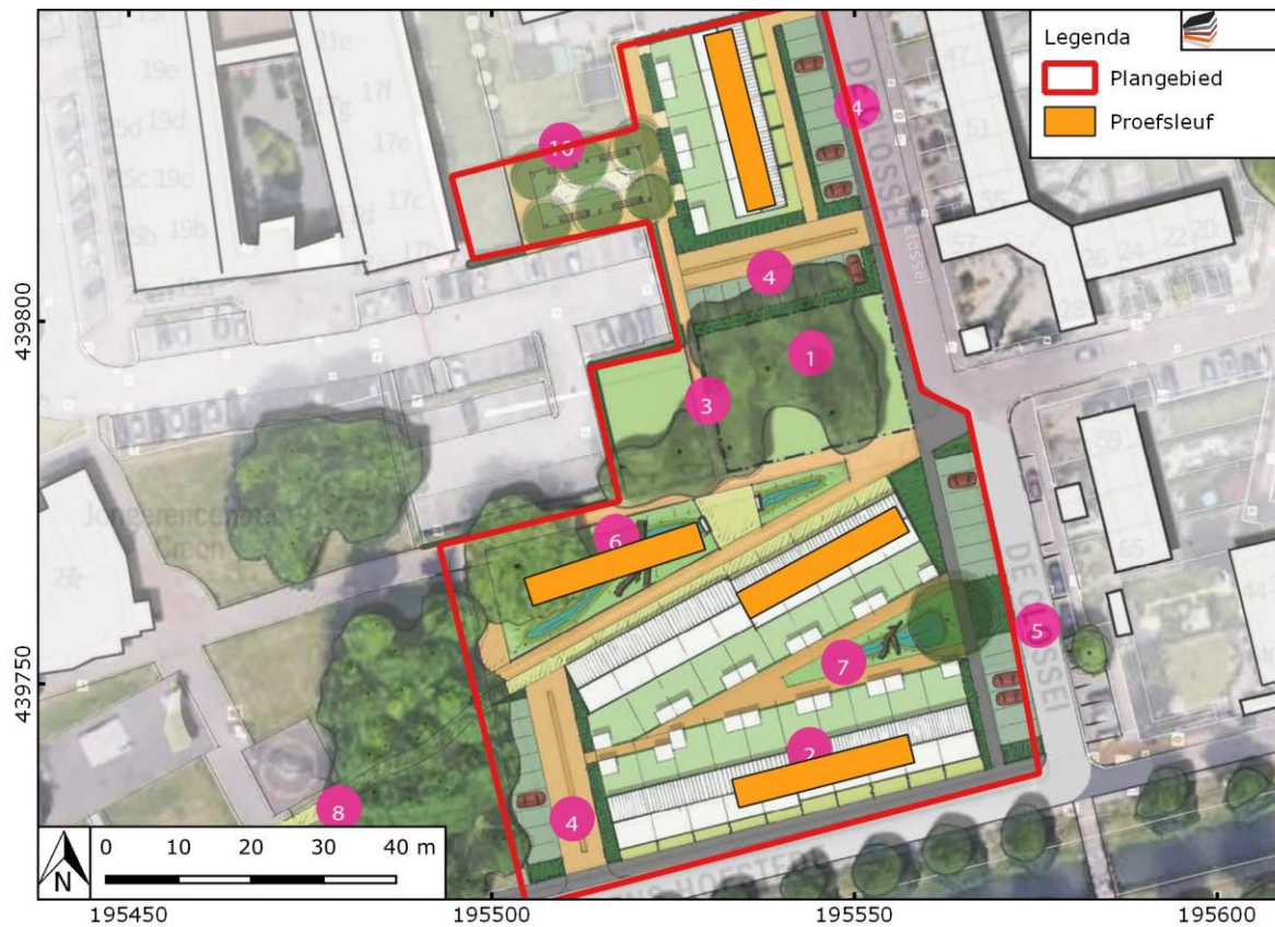
Indicatief puttenplan
