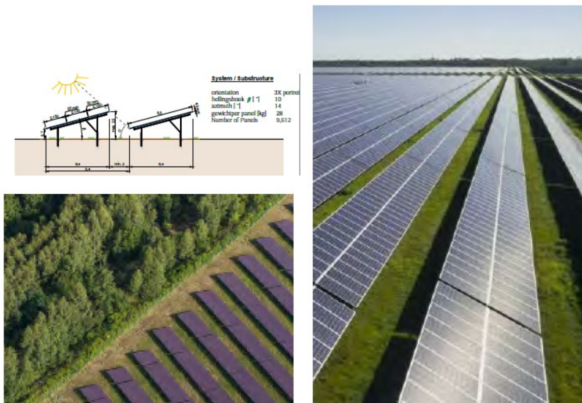
Figuur 6. Referentiebeelden panelen in zuid opstelling met ruimte voor beheer tussen de panelen
