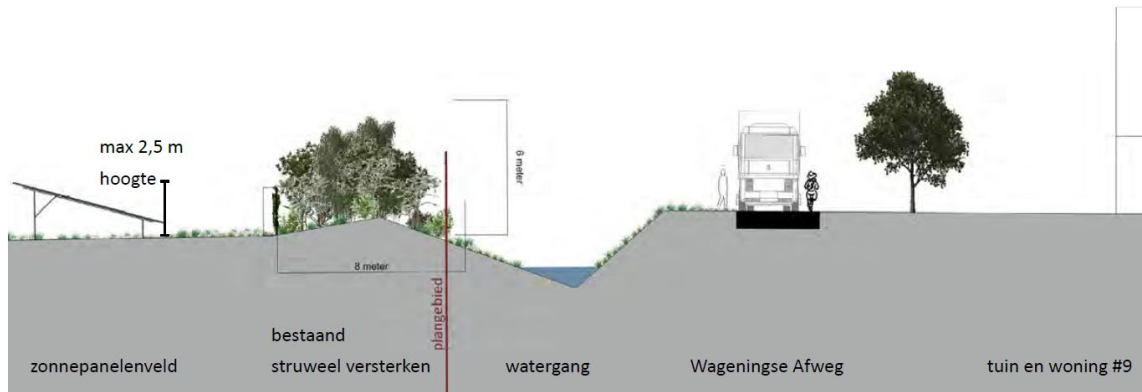
Figuur 19. Dwarsdoorsnede landschappelijke inpassing langs de Wageningse Afweg
