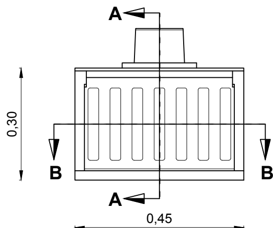
straatkolck 1-delig, type STR-9737 met ES vergrendeling
