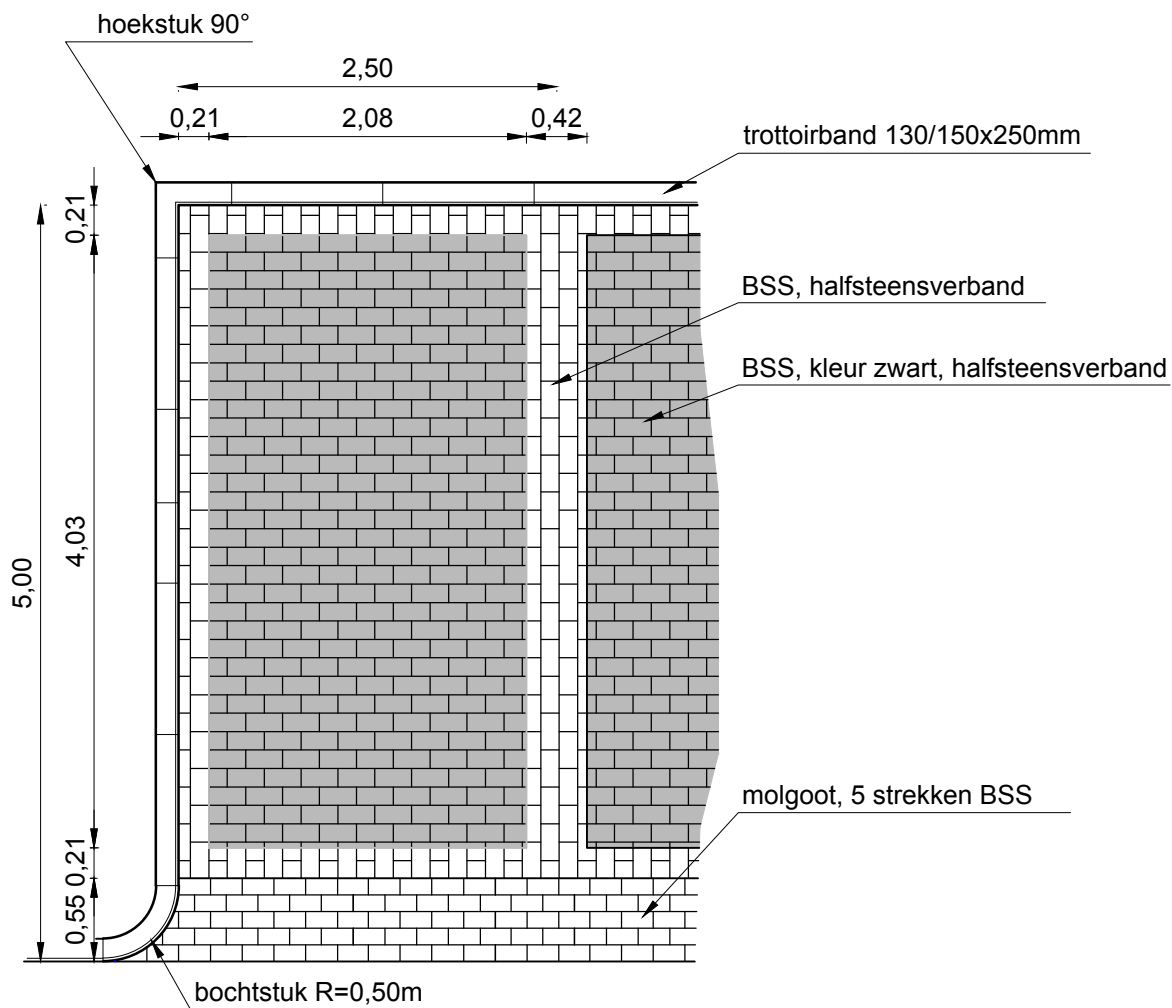
Bovenaanzicht
