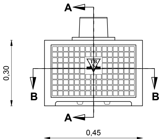
trottoirkolk 1-delig, type TRK-4718 met ES vergrendeling
