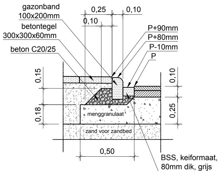
Detail gazonband langs fietspad met trottoir schaal 1:20
