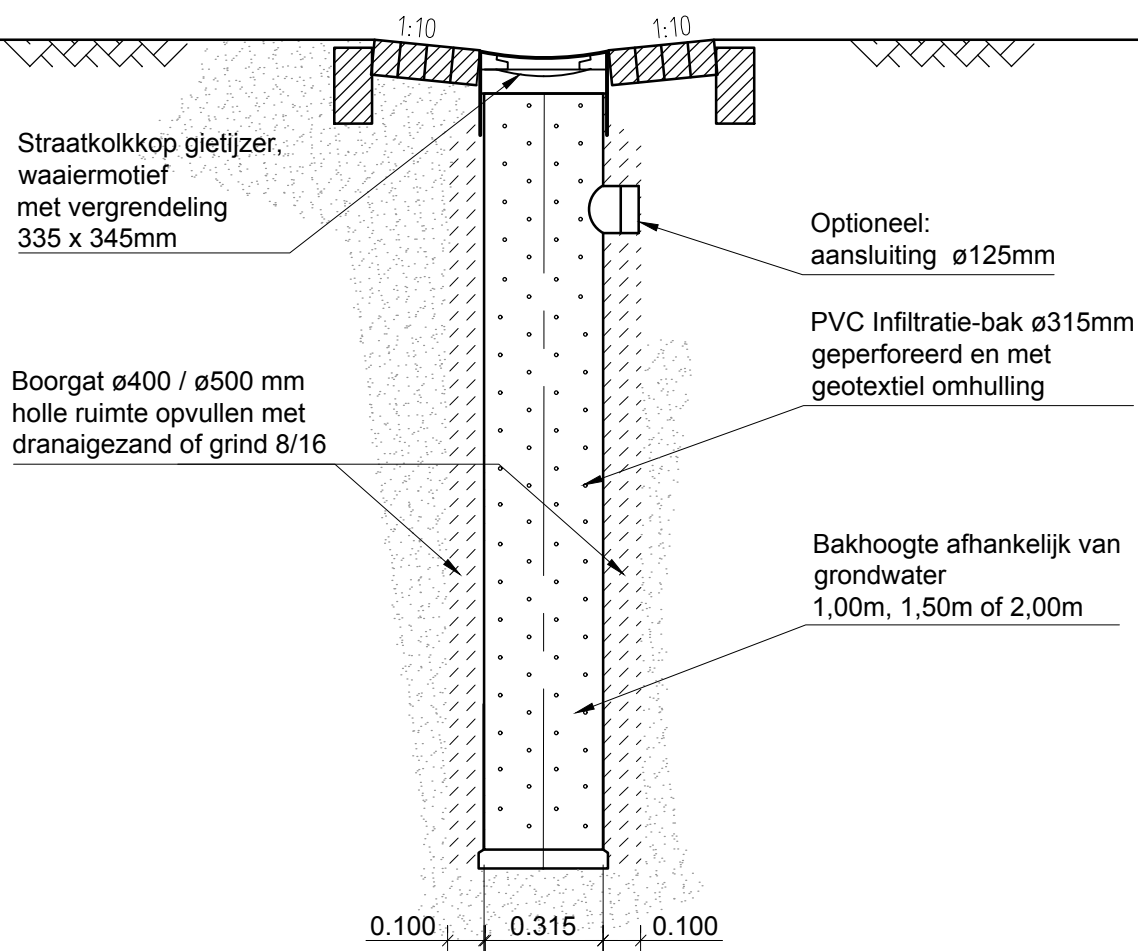
DOORSNEDE A-A
