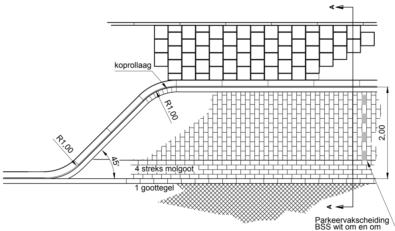
Bovenaanzicht langsparkeren
