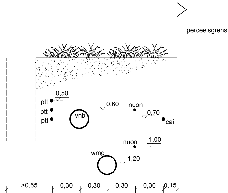
Weg met berm
