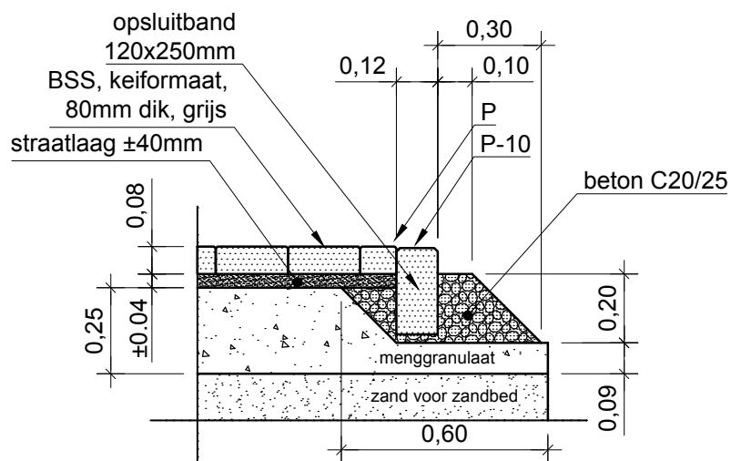
Detail kantopsluiting inrit schaal 1:20 (zwaar belaste inrit)
