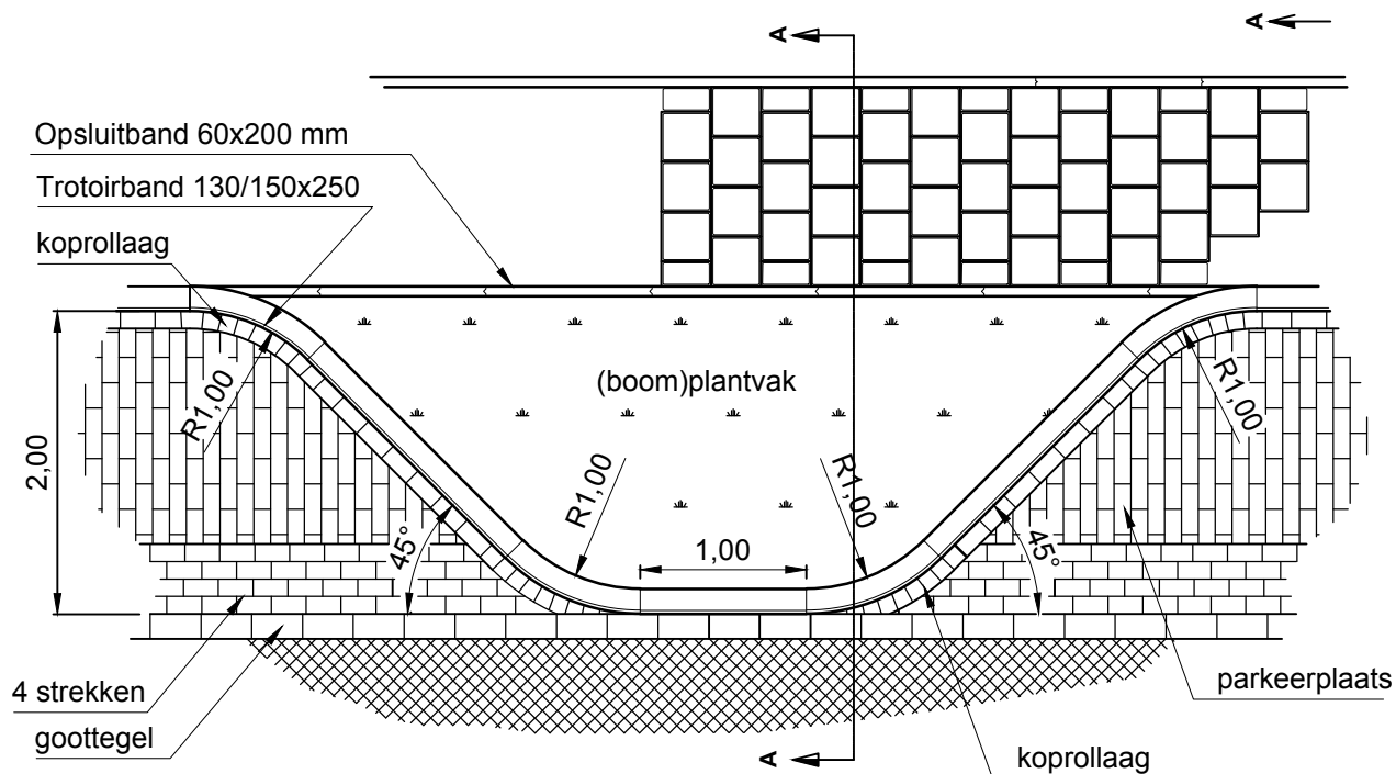
Bovenaanzicht boomplantvak in parkeerplaats
