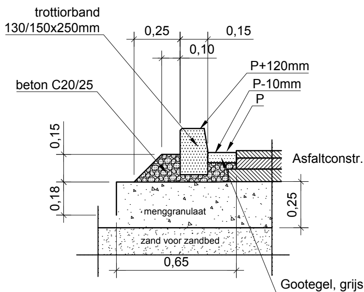
Detail trottoirband langs asfaltverharding schaal 1:20
