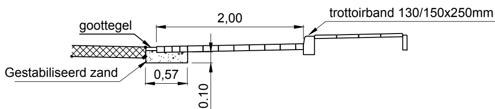
Doorsnede A-A
