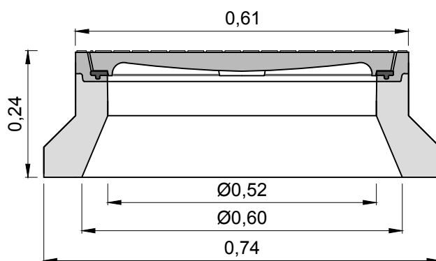
Dsn A-A
