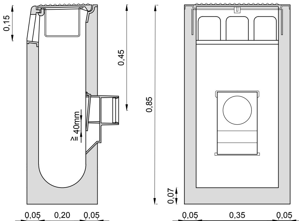
Dsn A-A
