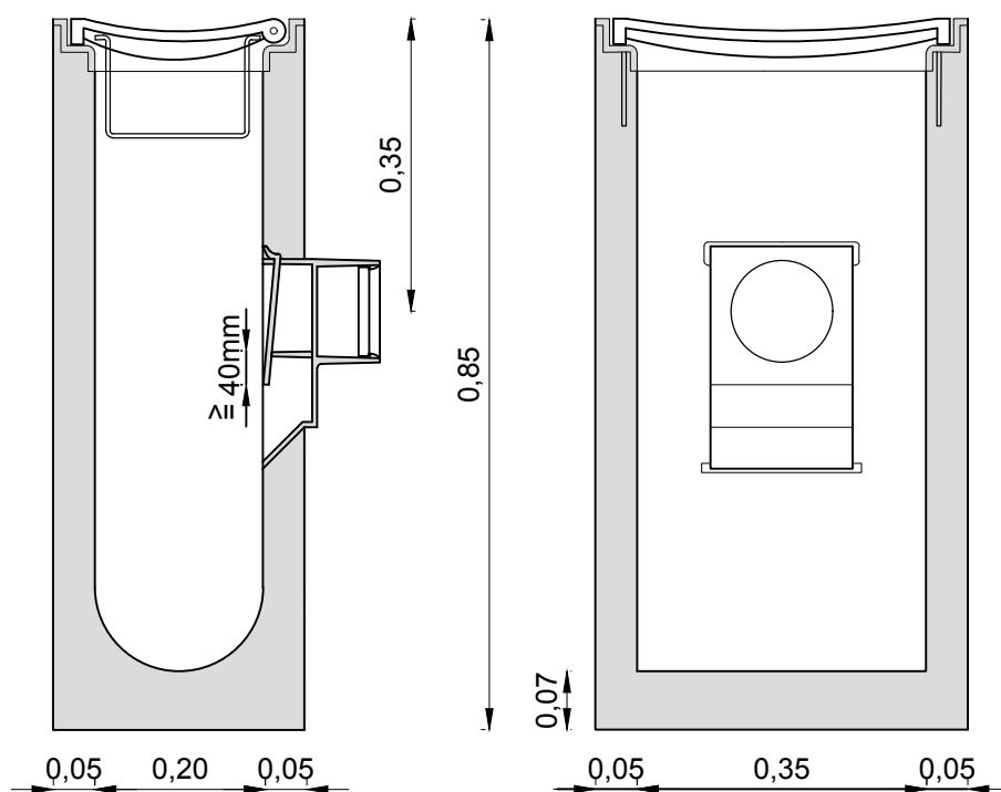
Dsn A-A
