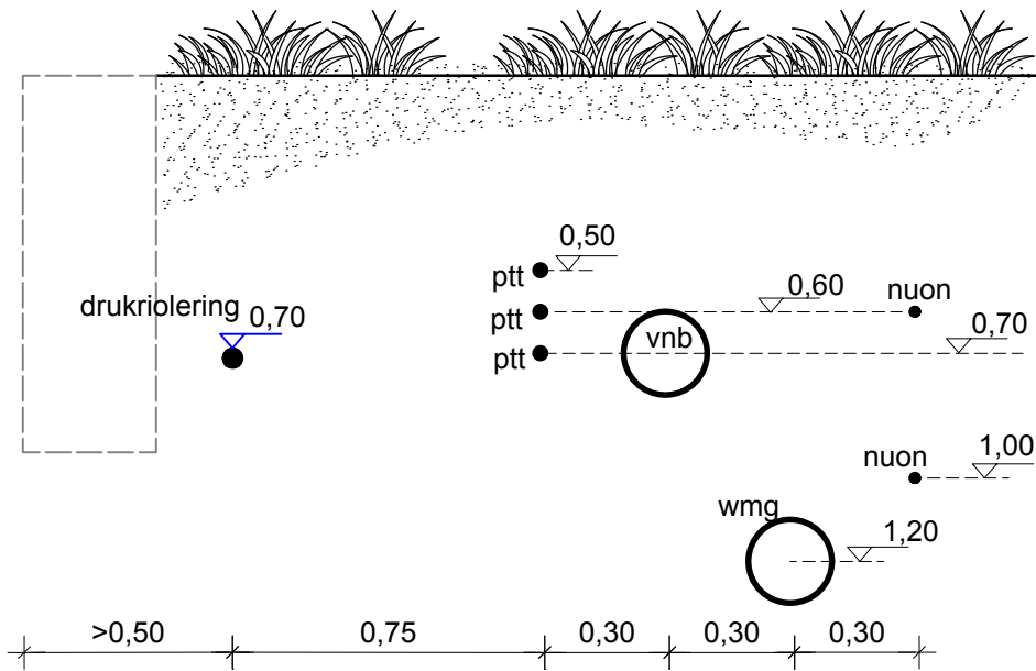
Weg zonder bermsloot
