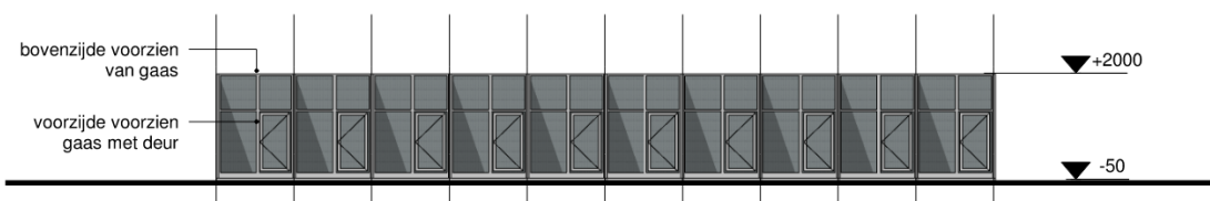
Afbeelding 6 - Gevelaanzicht volières
