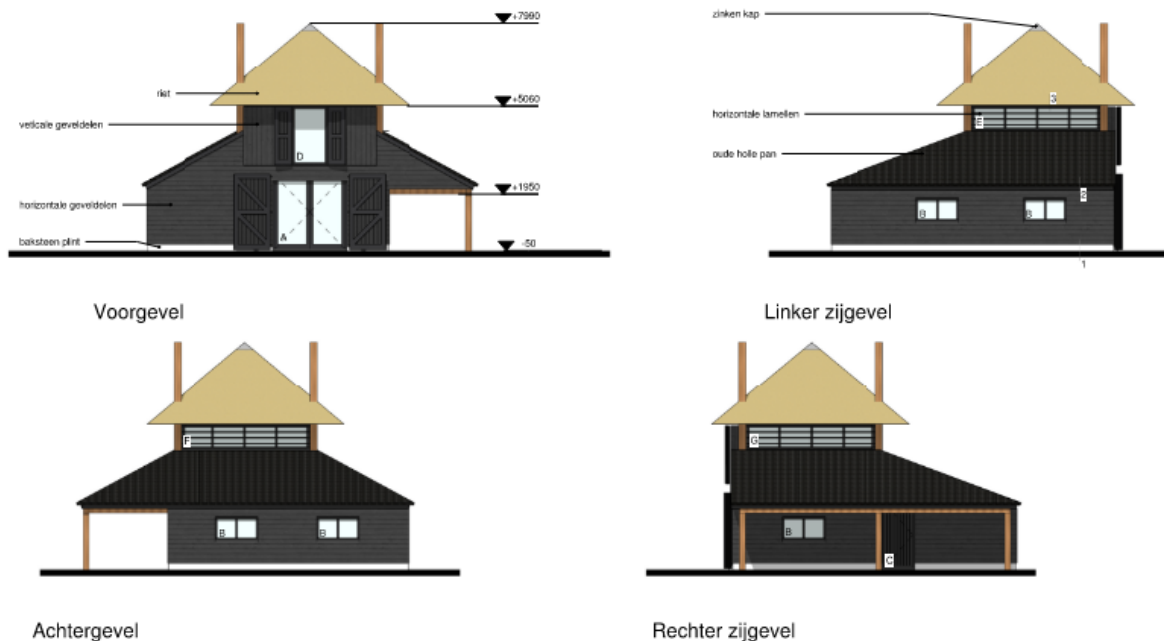
Afbeelding 3 - Gevelaanzichten steltenberg
