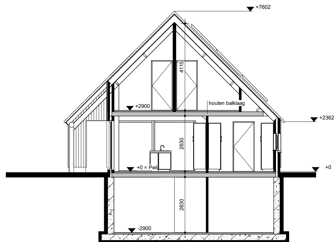
Doorsnede A-A
