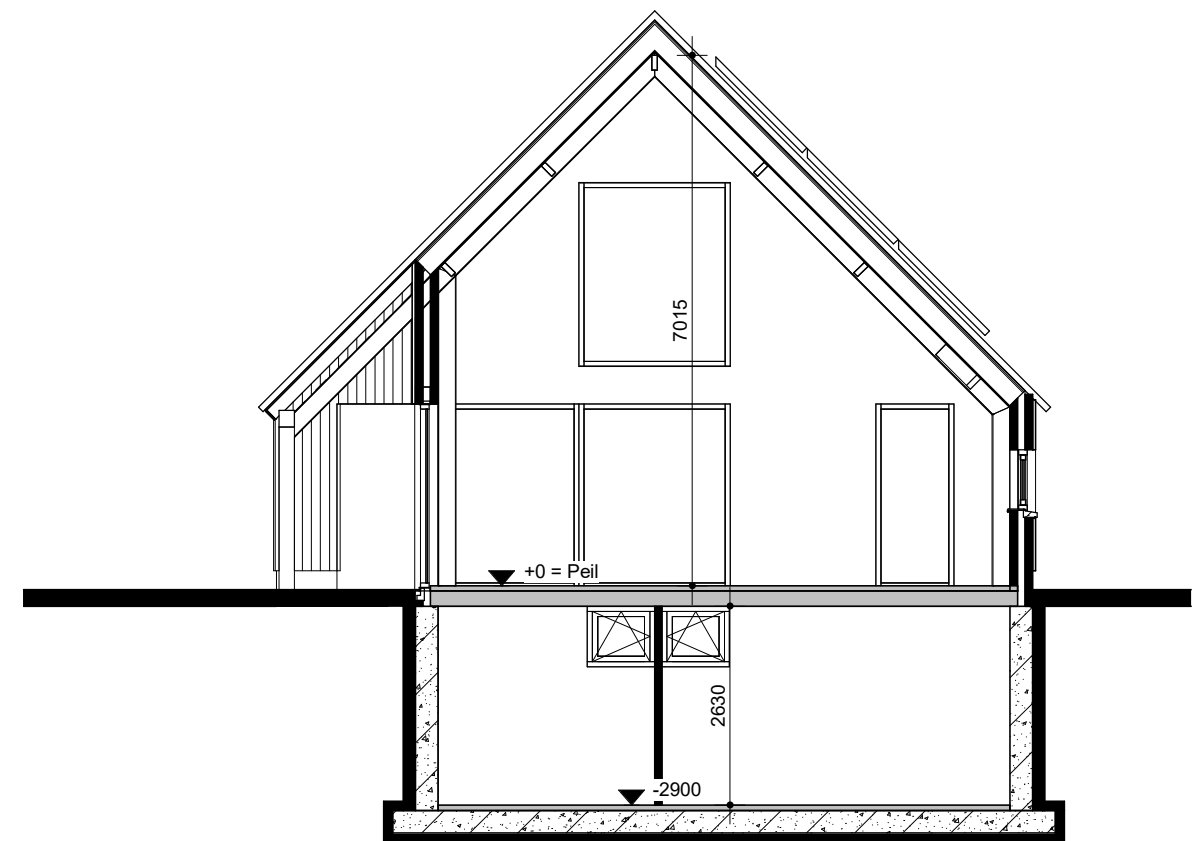
Doorsnede B-B
