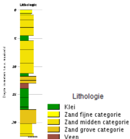
Afbeelding 2.1: Boorprofiel
