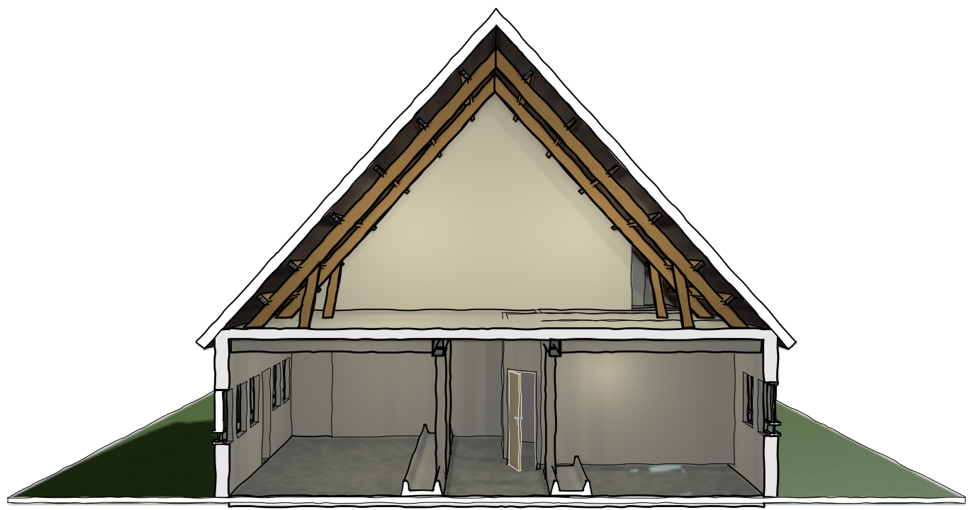
Dwarsdoorsnede bestaand
