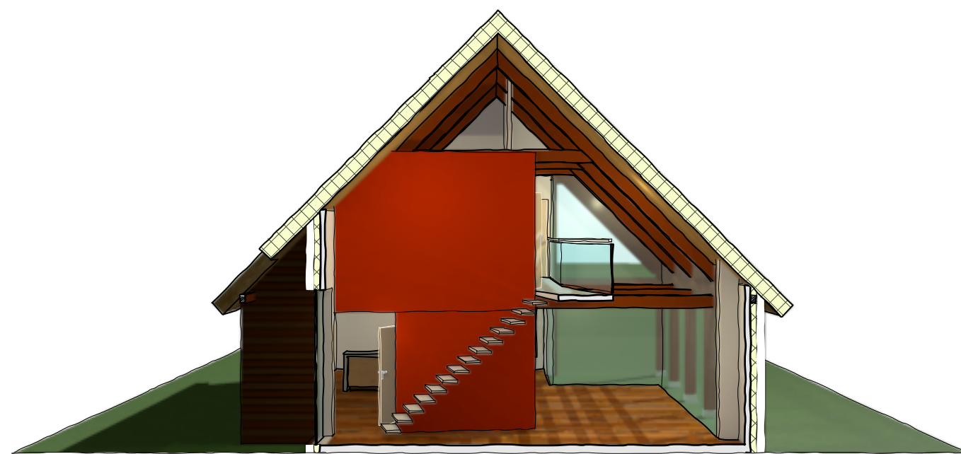
Dwarsdoorsnede
