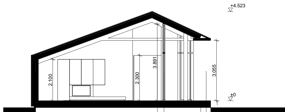
Doorsnede B-B
