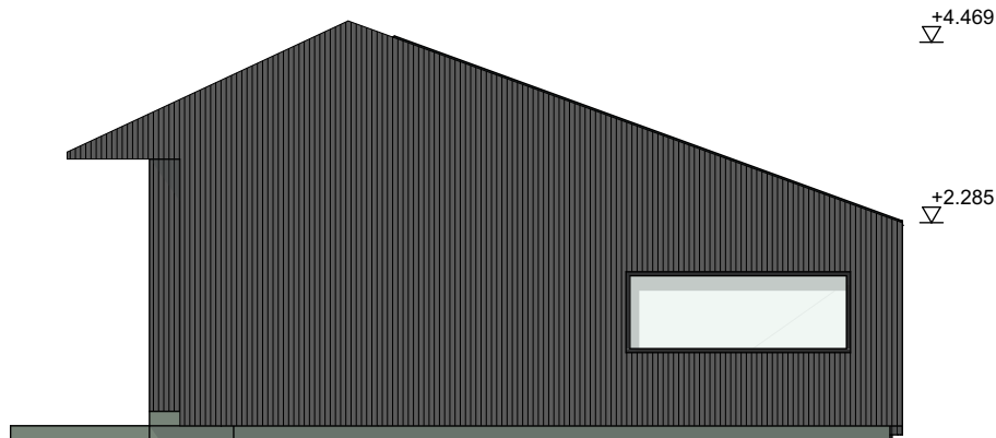
Rechtergevel
