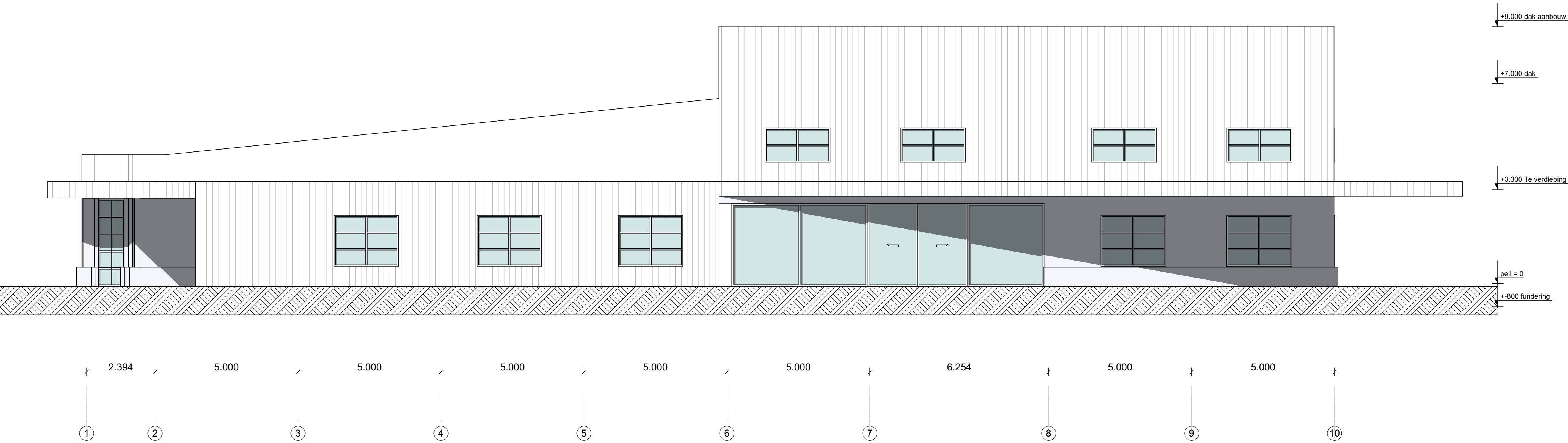
Rechterzijgevel
