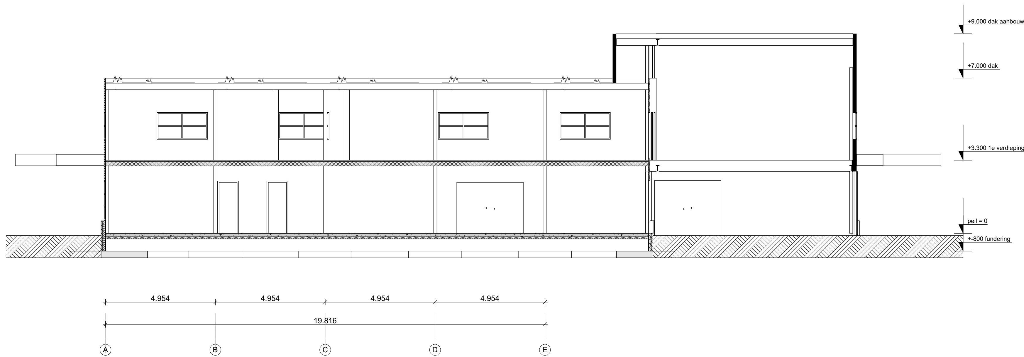
Doorsnede A-A
