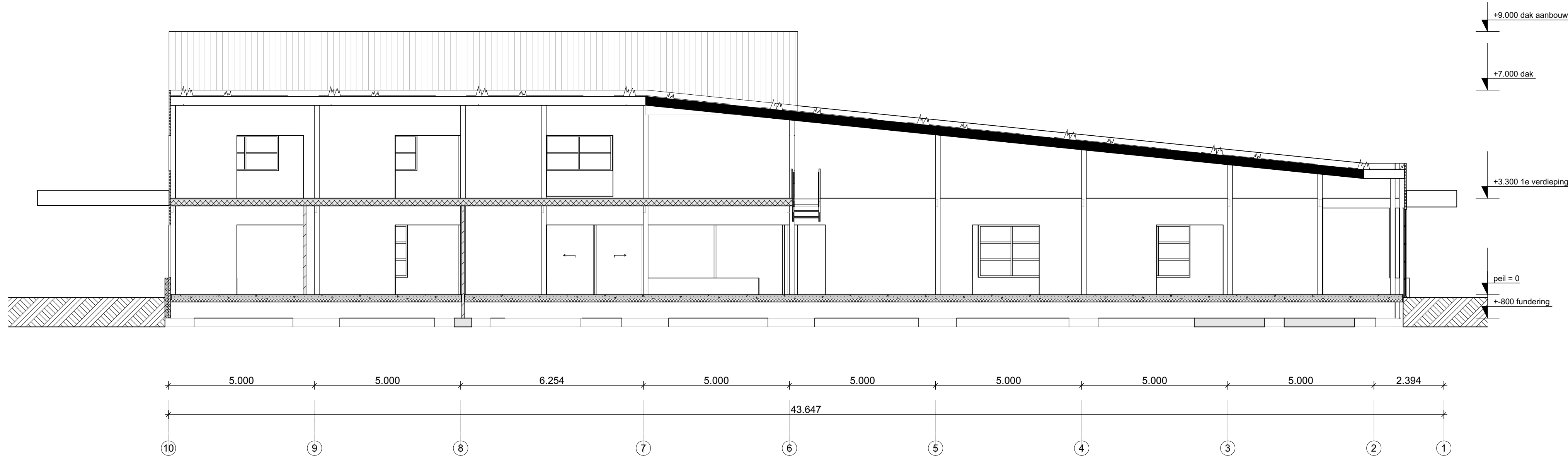
Doorsnede B-B
