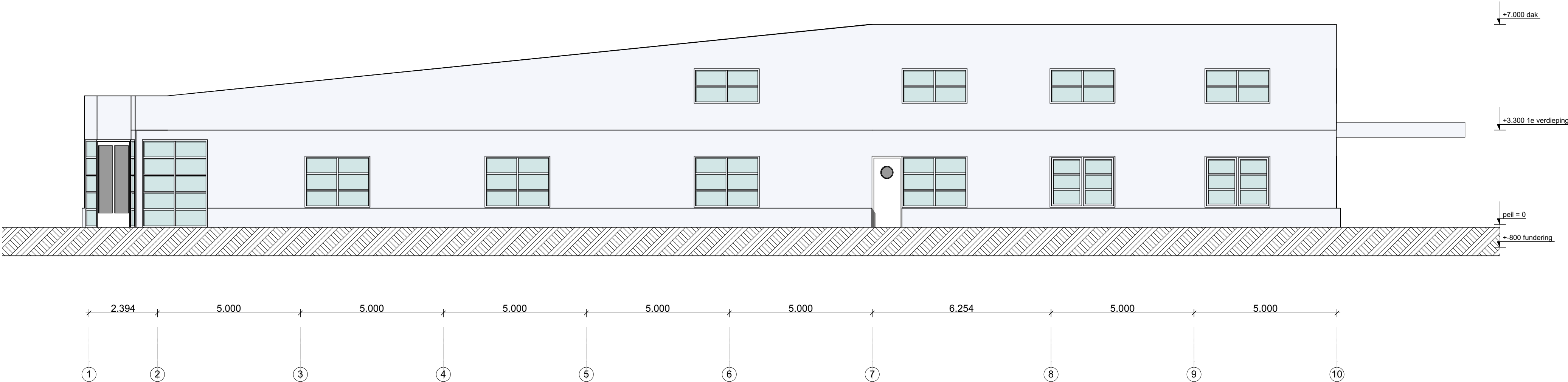
Rechterzijgevel
