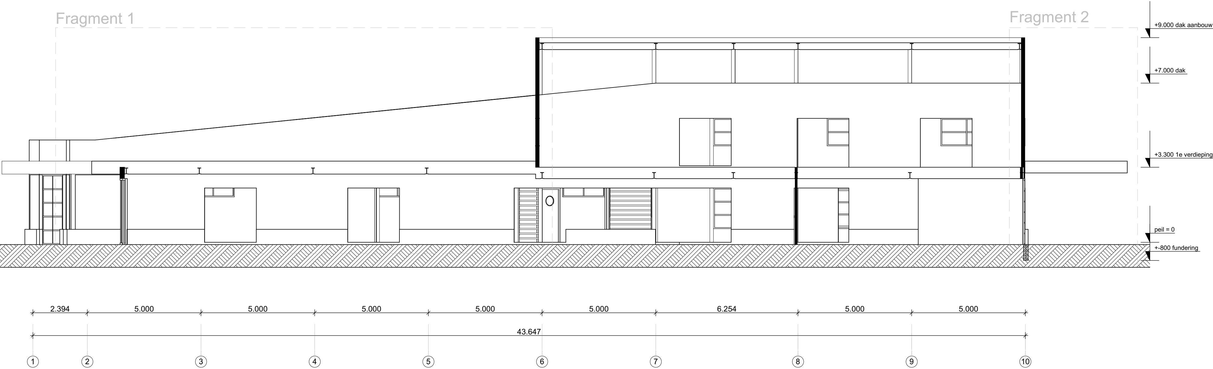
Doorsnede C-C
