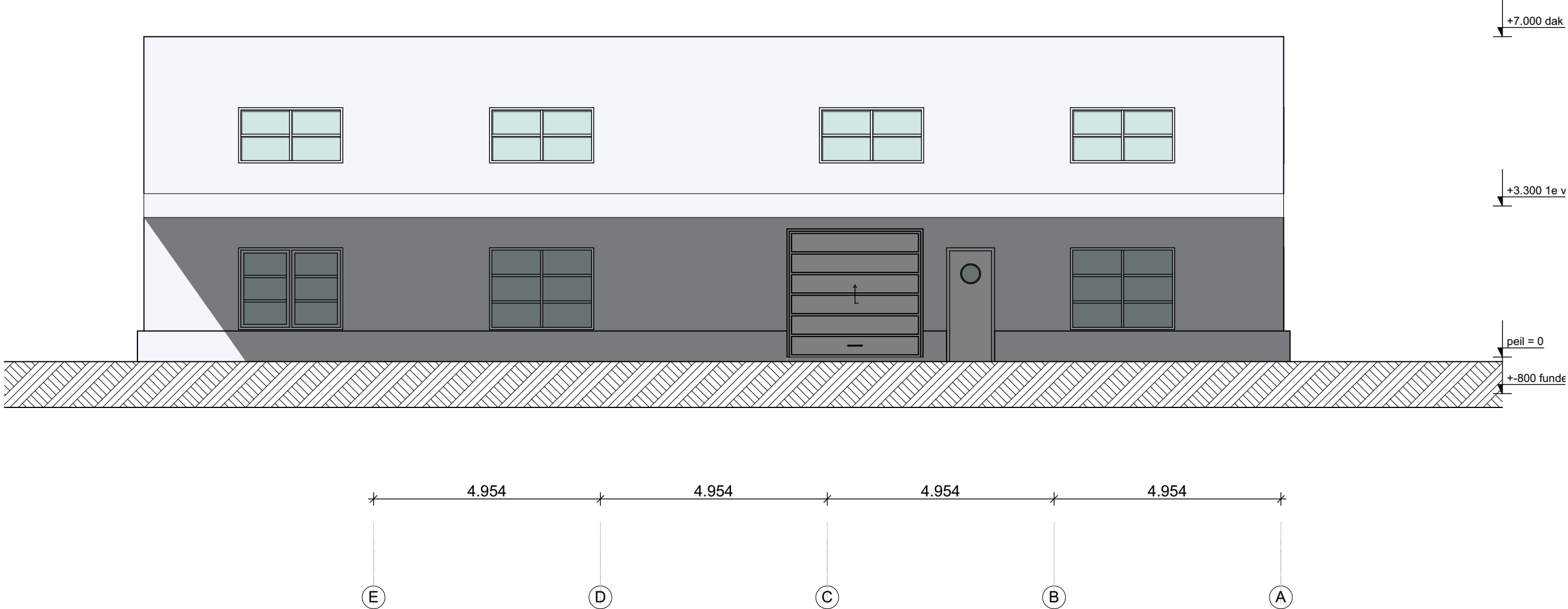
Achtergevel
