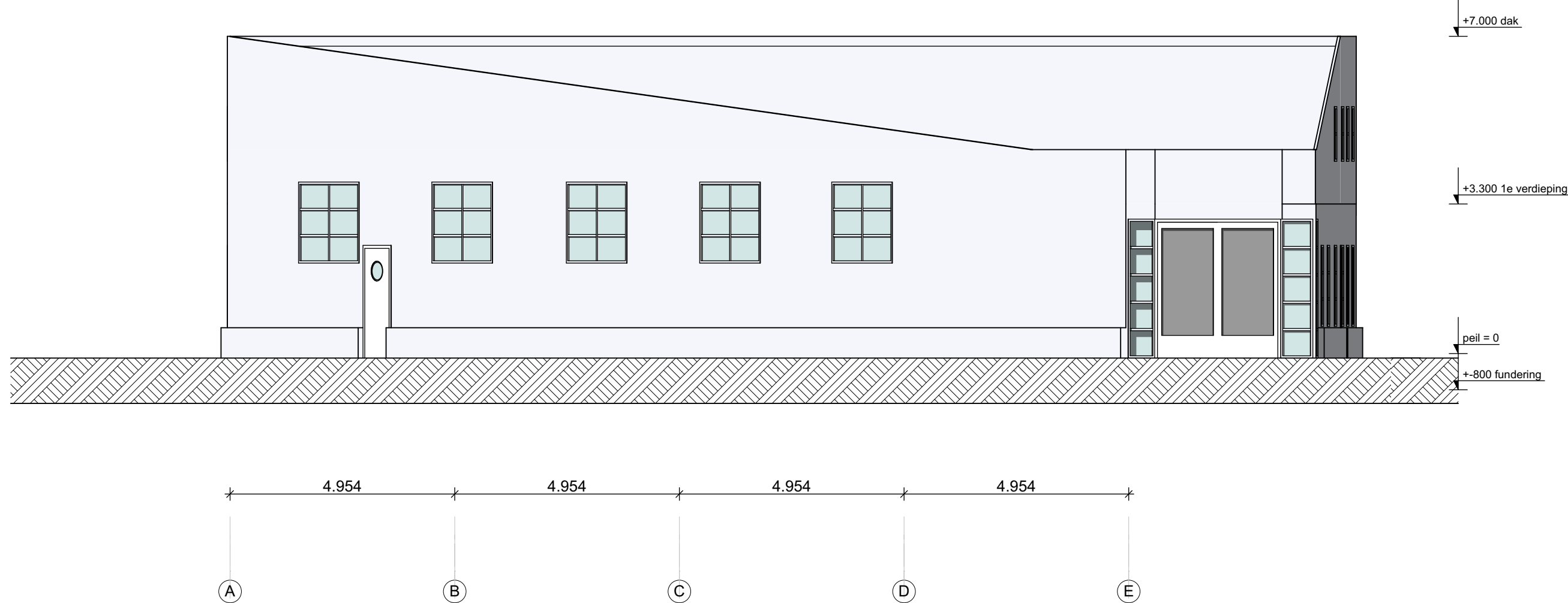
Voorgevel
