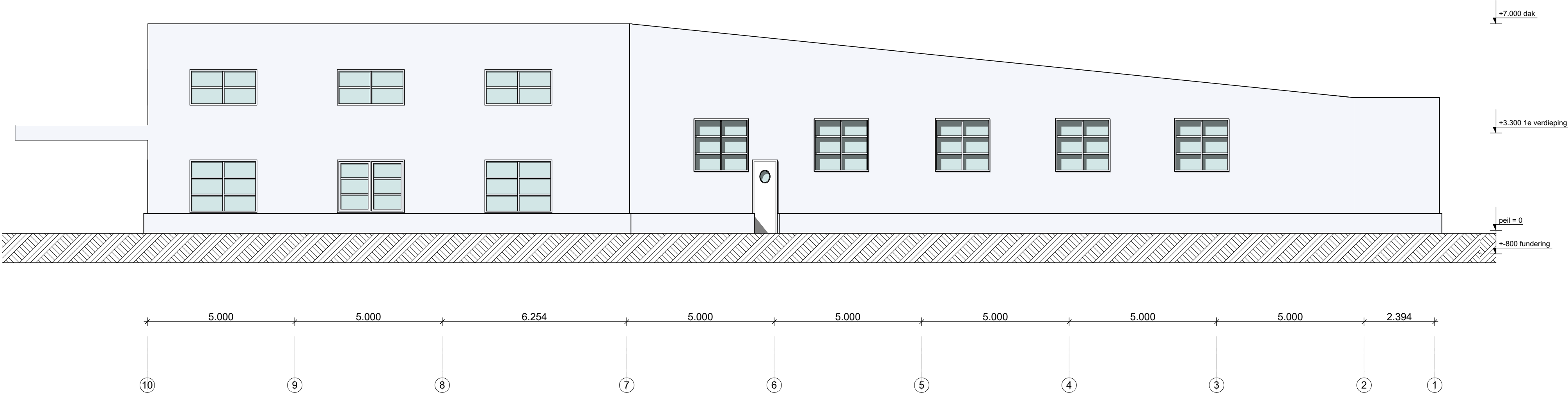
Linkerzijgevel
