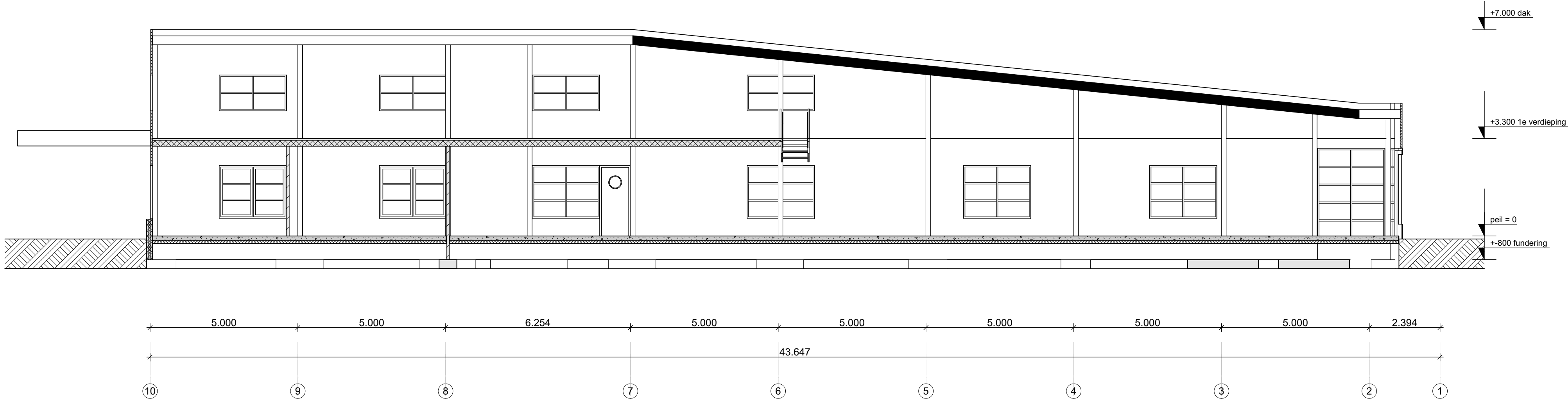
Doorsnede B-B
