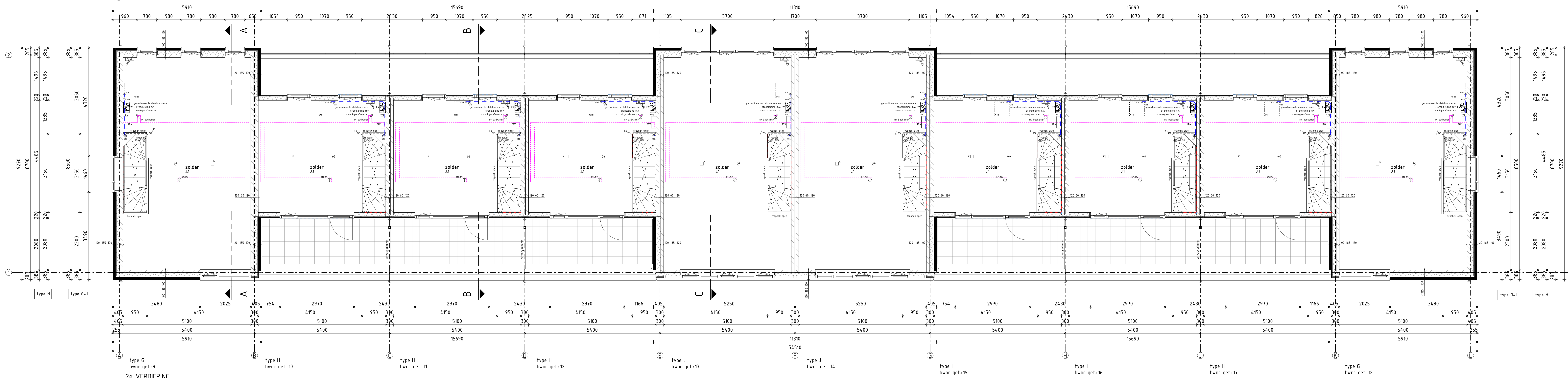
2e VERDIEPING
