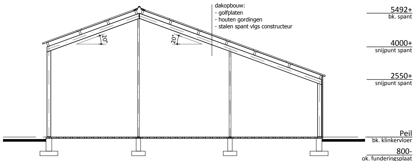
doorsnede A-A
