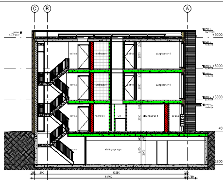
doorsnede BB
