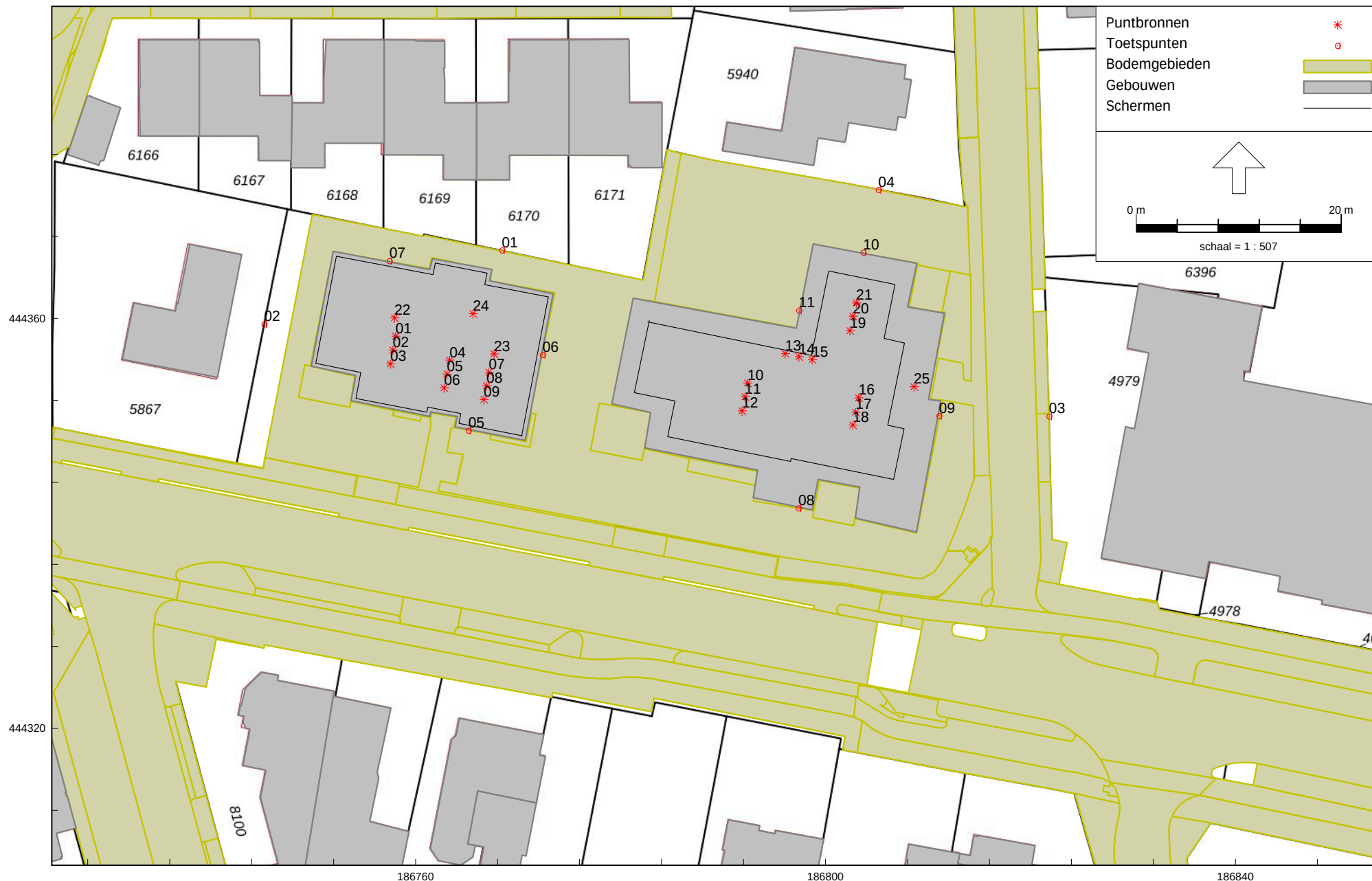
Overzicht van het rekenmodel met de ligging van de ingevoerde objecten, geluidbronnen en rekenpunten
