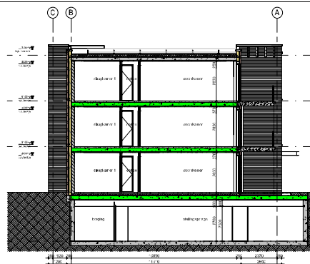
doorsnede AA
