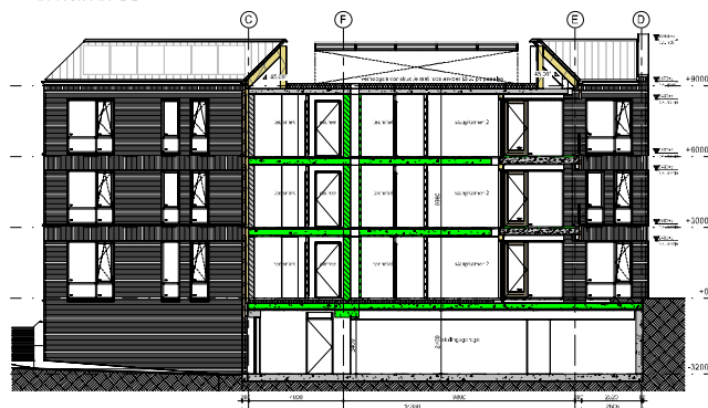
doorsnede EE
