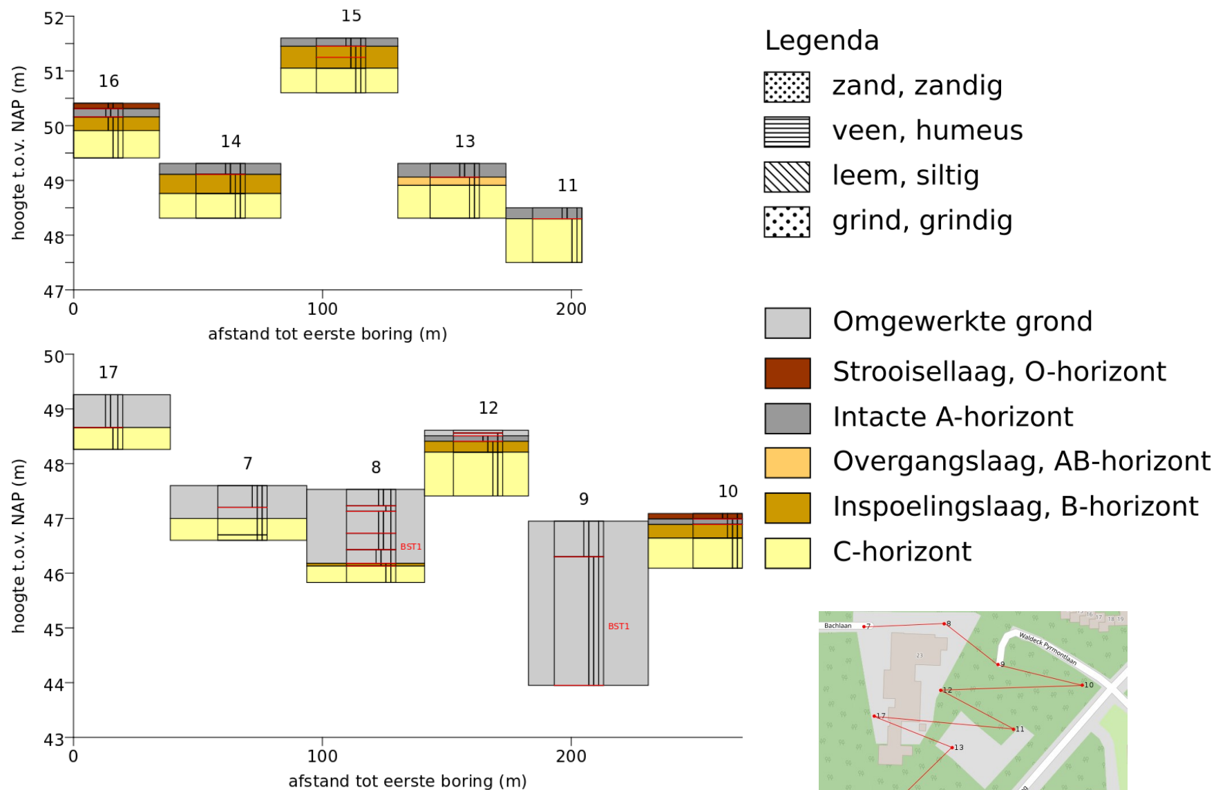
Figuur 34: Schematische weergave van boorprofielen in deelgebied A.
