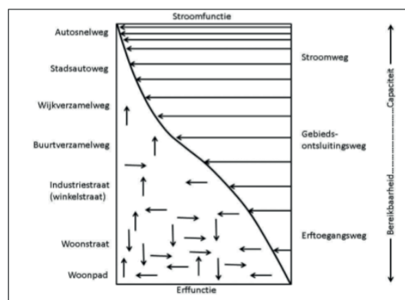
Figuur 4.2: Schematische weergave van verschillende soorten wegen
