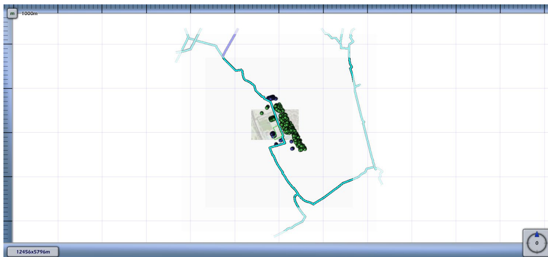
4.4 Figuur 4.4 Groepsrisico screening voor 7260_leiding-N-576-67-deel-1 van N.V. Nederlandse Gasunie
