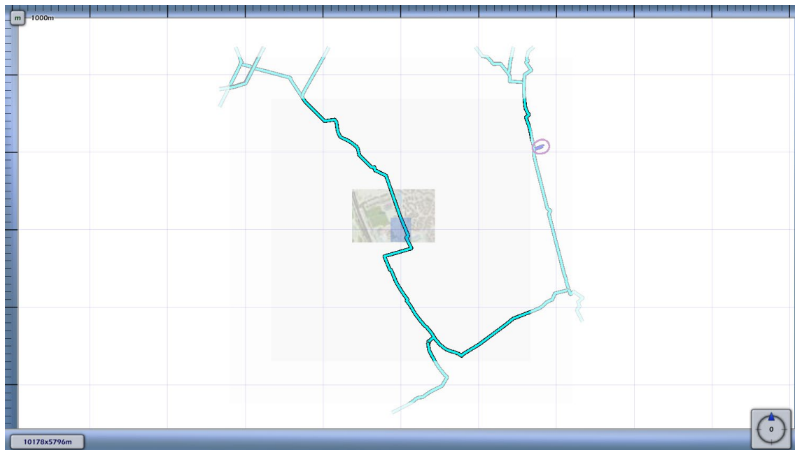
3.8 Figuur 3.8 Plaatsgebonden risico voor 7260_leiding-N-576-70-deel-1 van N.V. Nederlandse Gasunie
