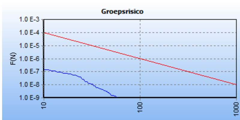
5.8 Figuur 5.8 FN curve voor 7260_leiding-N-576-70-deel-1 van N.V. Nederlandse Gasunie voor de kilometer tussen stationing 2660.00 en stationing 3660.00
