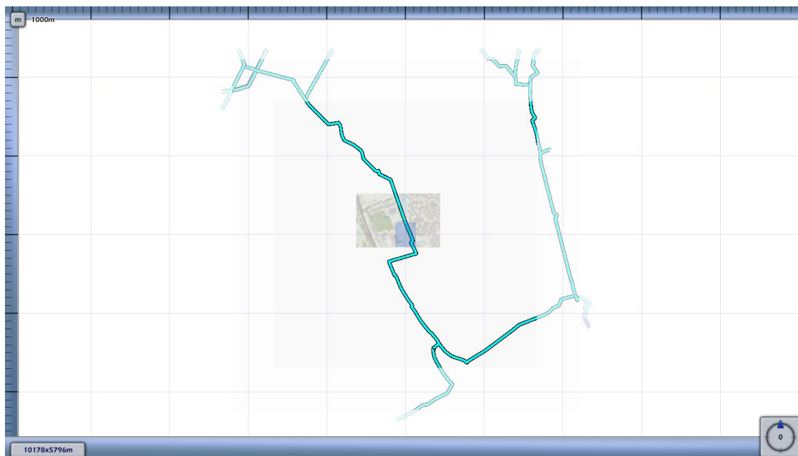
3.12 Figuur 3.12 Plaatsgebonden risico voor 7260_leiding-N-576-77-deel-1 van N.V. Nederlandse Gasunie
