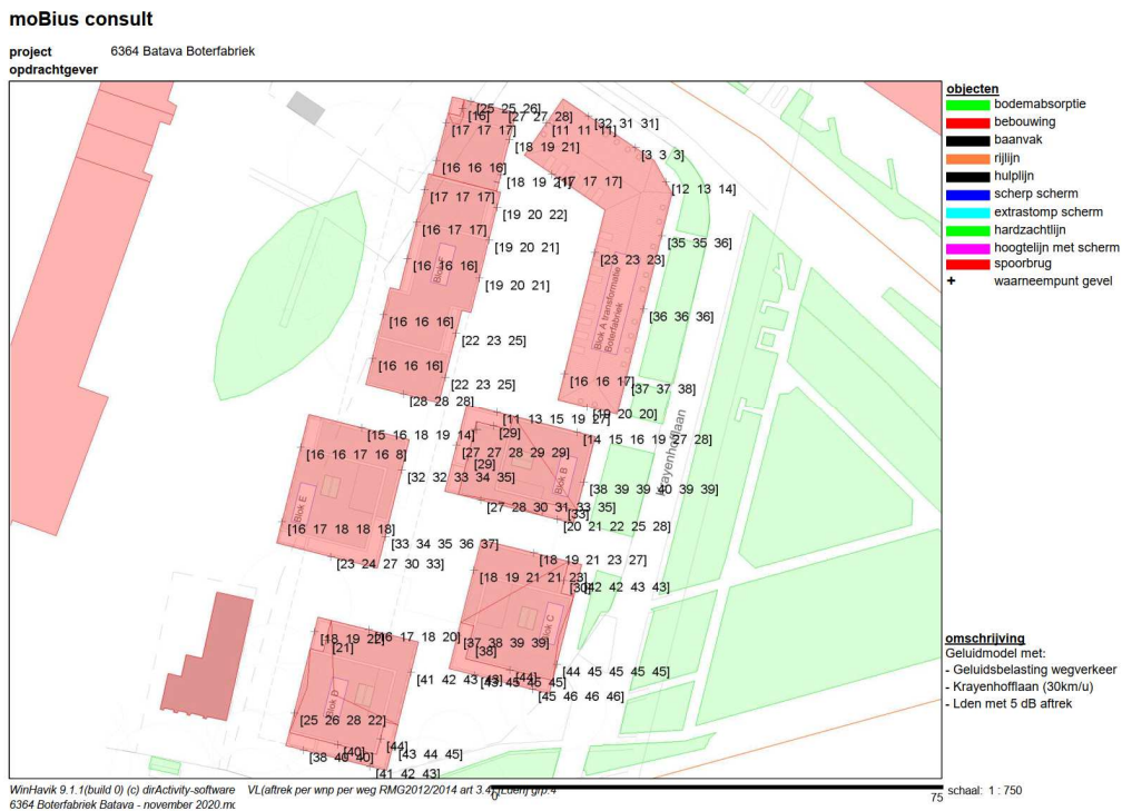
Figuur 8: Geluidsbelasting wegverkeer Krayenhofflaan (30 km/u), Lden met 5 dB aftrek
