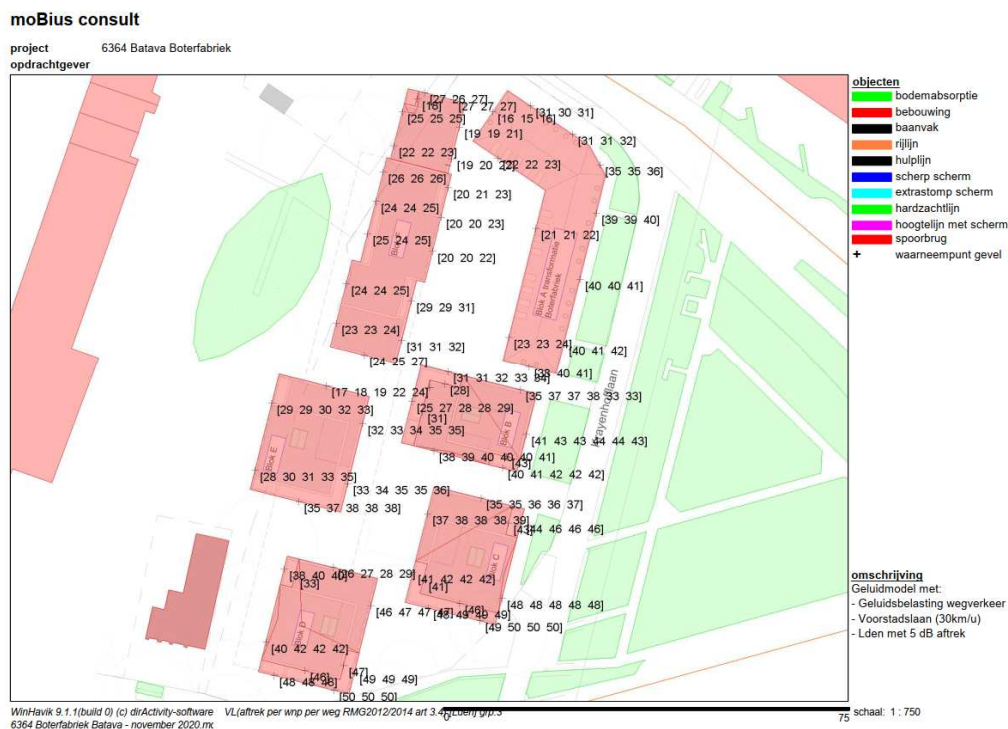
Figuur 7: Geluidsbelasting wegverkeer Voorstadslaan (30 km/u), Lden met 5 dB aftrek
