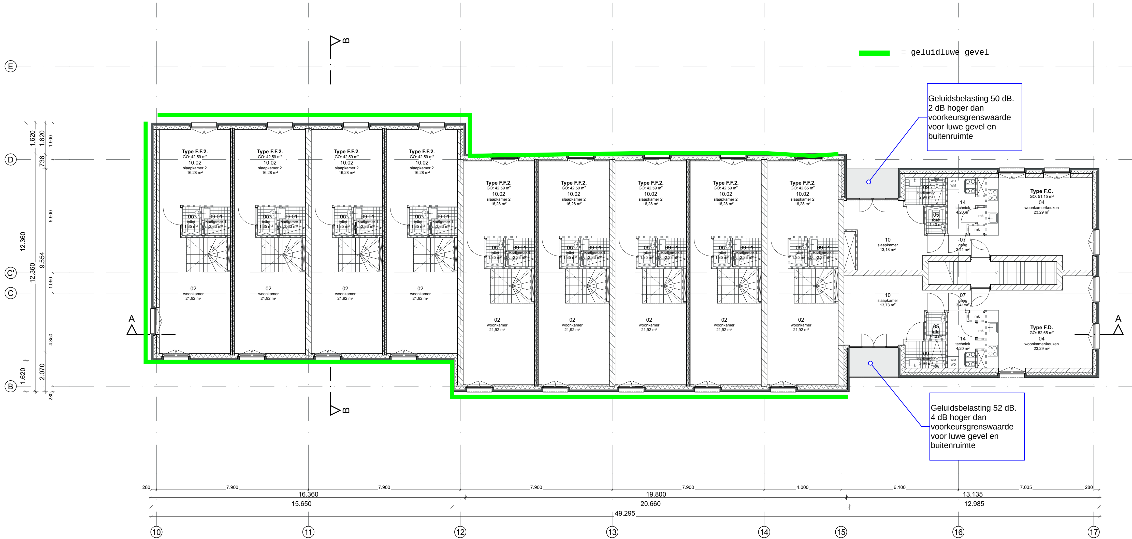
EERSTE VERDIEPING (3.200+P)
