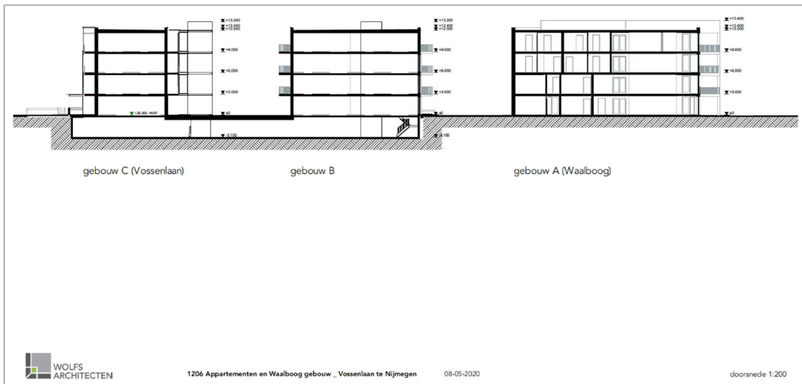
Afb. 5. Dwarsdoorsnede van de nieuwbouw in het plangebied (bron: Wolfs Architecten).
