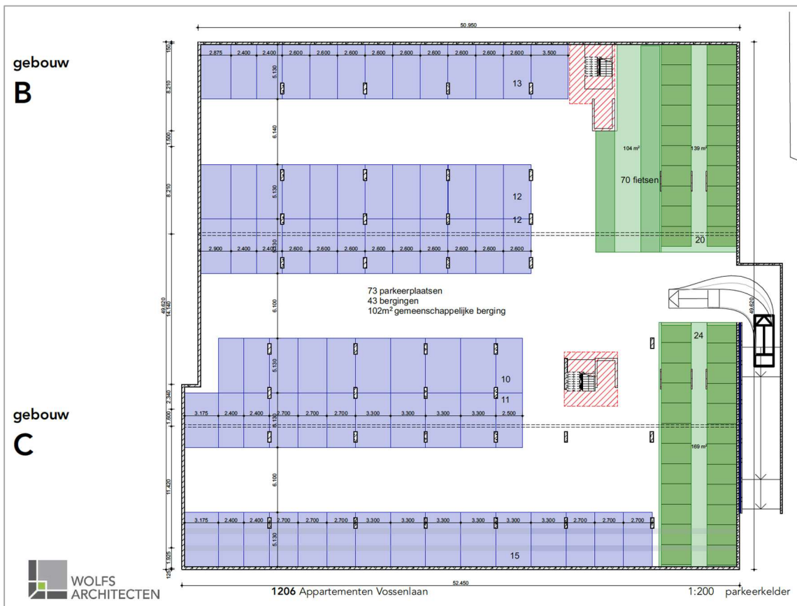
Afb. 6. Toekomstige situatie van de parkeerkelder onder gebouwen B en C in het plangebied (bron: Wolfs Architecten).
