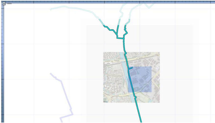
3.5 Figuur 3.5 Plaatsgebonden risico voor 8194_leiding-N-576-70-deel-1 van N.V. Nederlandse Gasunie
