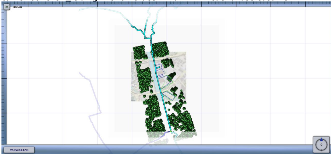
Figuur 4.5 Kilometer leiding behorende bij de maximale overschrijding van de FN-curve voor 8194_leiding-N-576-70-deel-1 van N.V. Nederlandse Gasunie
