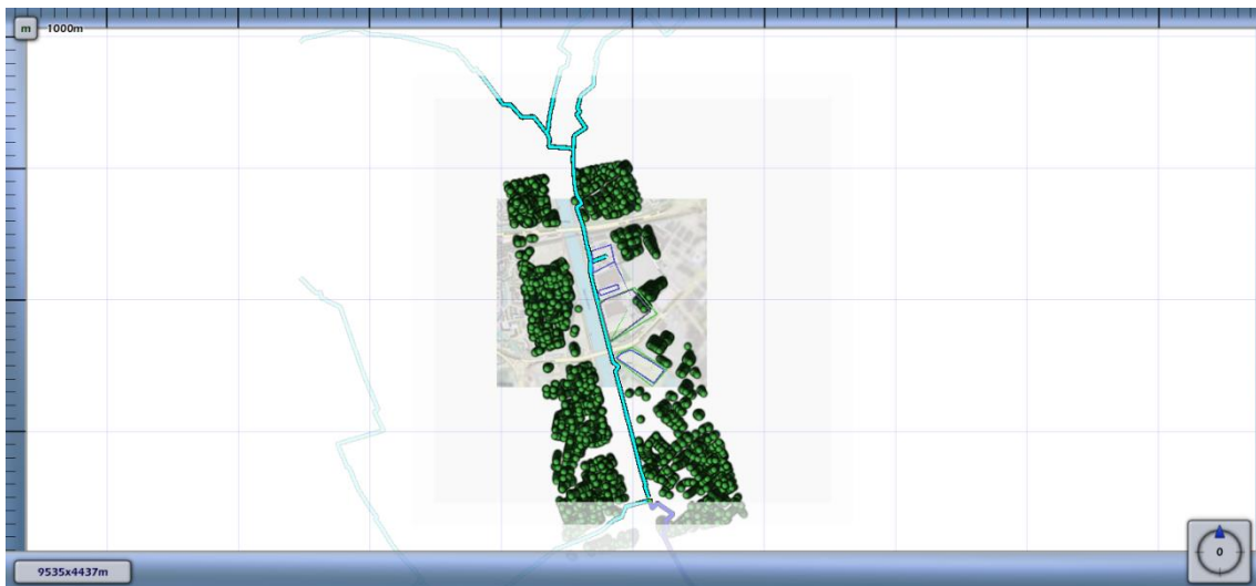
4.7 Figuur 4.7 Groepsrisico screening voor 8194_leiding-N-576-75-deel-1 van N.V. Nederlandse Gasunie
