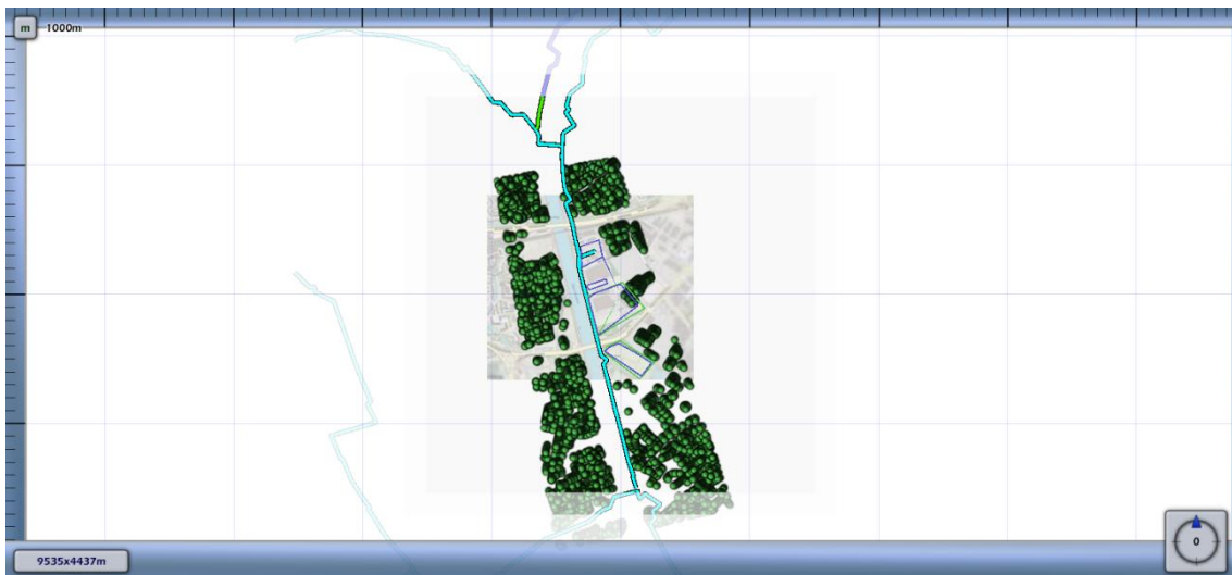
4.4 Figuur 4.4 Groepsrisico screening voor 8194_leiding-N-576-69-deel-1 van N.V. Nederlandse Gasunie
