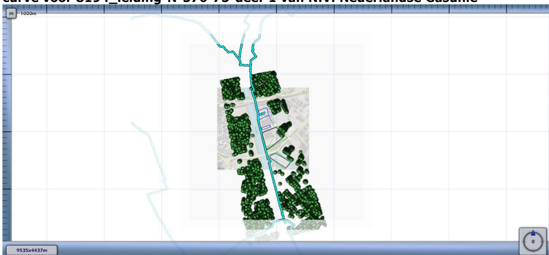
Figuur 4.7 Kilometer leiding behorende bij de maximale overschrijding van de FN-curve voor 8194_leiding-N-576-75-deel-1 van N.V. Nederlandse Gasunie
