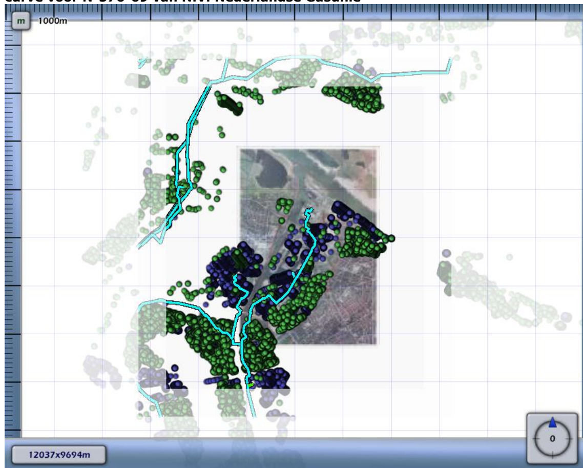
Figuur 4.11 Kilometer leiding behorende bij de maximale overschrijding van de FN-curve voor N-576-69 van N.V. Nederlandse Gasunie
