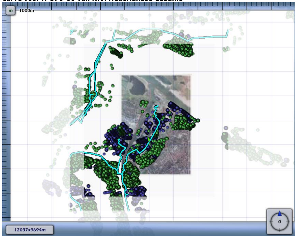
Figuur 4.8 Kilometer leiding behorende bij de maximale overschrijding van de FN-curve voor N-576-66 van N.V. Nederlandse Gasunie
