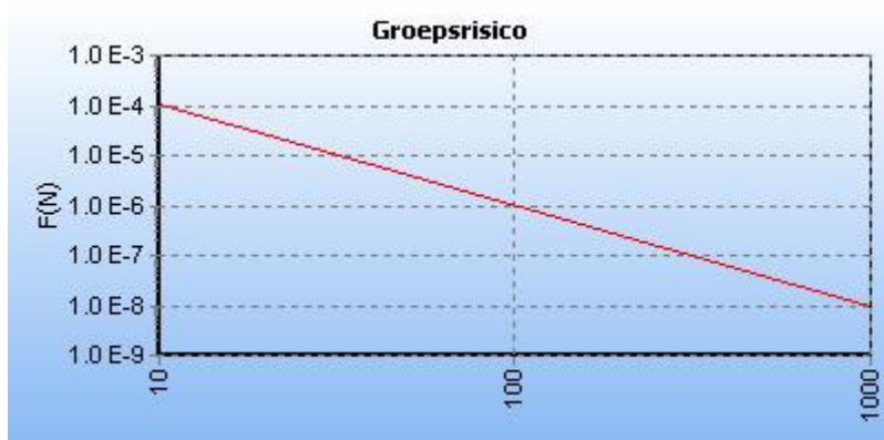
5.11 Figuur 5.11 FN curve voor N-576-69 van N.V. Nederlandse Gasunie voor de kilometer tussen stationing 0.00 en stationing 110.00
