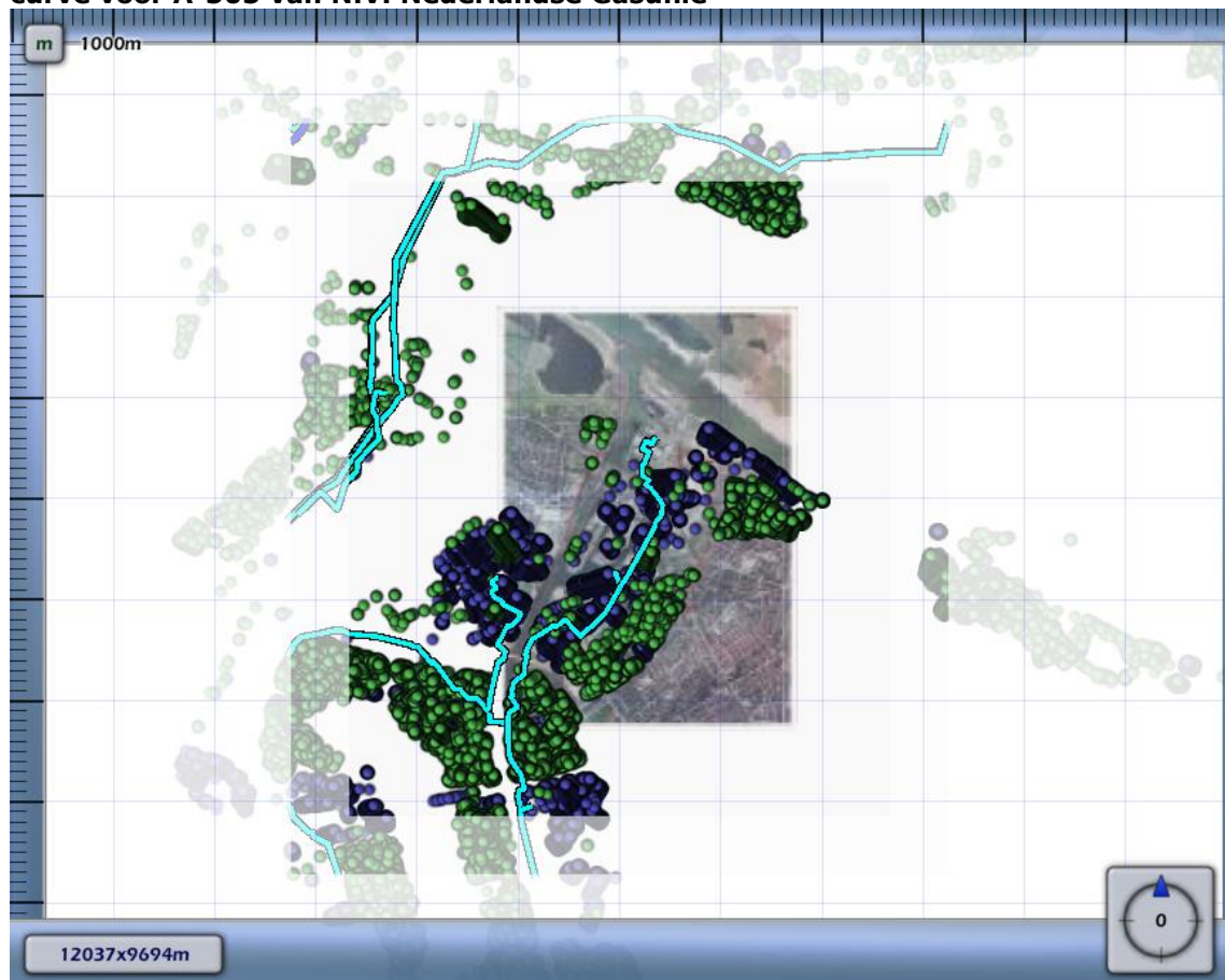
Figuur 4.1 Kilometer leiding behorende bij de maximale overschrijding van de FN-curve voor A-505 van N.V. Nederlandse Gasunie
