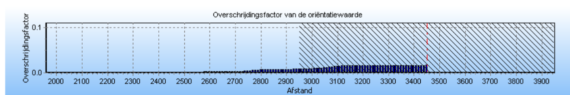
4.7 Figuur 4.7 Groepsrisico screening voor N-576-02 van N.V. Nederlandse Gasunie
