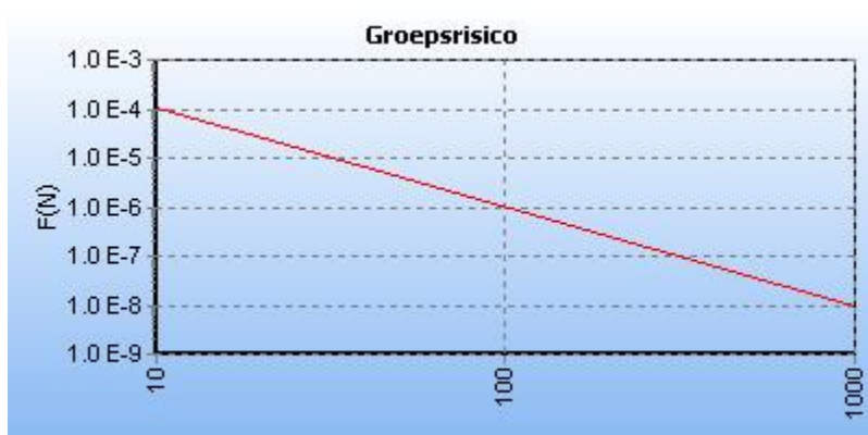
5.8 Figuur 5.8 FN curve voor N-576-66 van N.V. Nederlandse Gasunie voor de kilometer tussen stationing 0.00 en stationing 160.00
