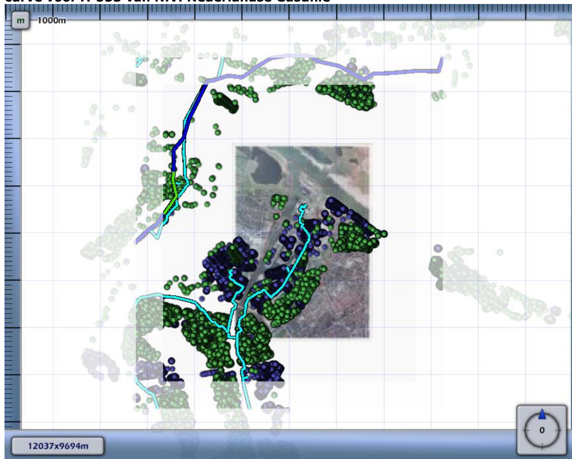
Figuur 4.4 Kilometer leiding behorende bij de maximale overschrijding van de FN-curve voor A-533 van N.V. Nederlandse Gasunie
