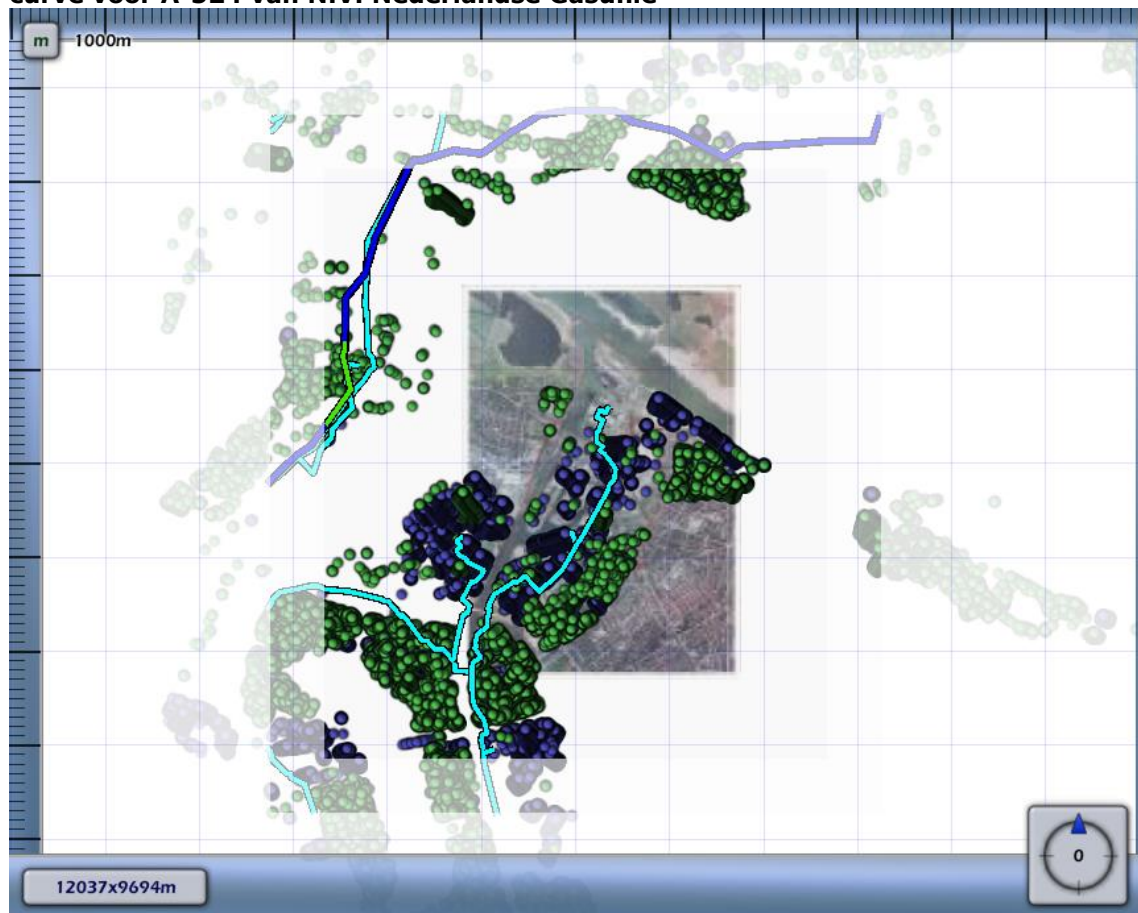
Figuur 4.3 Kilometer leiding behorende bij de maximale overschrijding van de FN-curve voor A-524 van N.V. Nederlandse Gasunie
