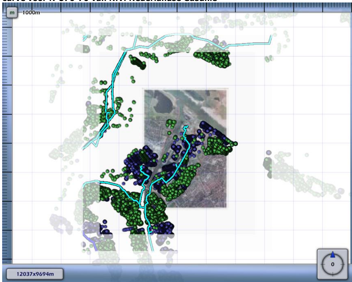
Figuur 4.12 Kilometer leiding behorende bij de maximale overschrijding van de FN-curve voor N-576-70 van N.V. Nederlandse Gasunie
