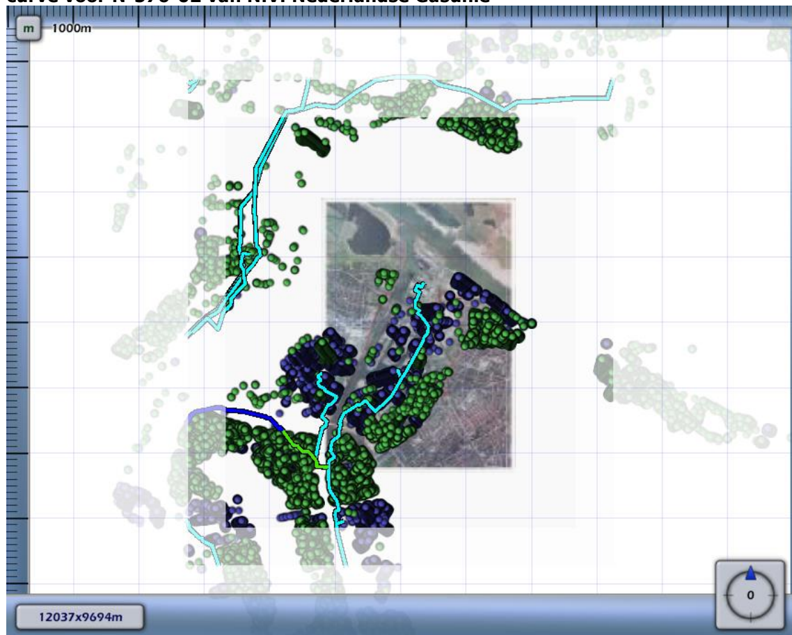
Figuur 4.7 Kilometer leiding behorende bij de maximale overschrijding van de FN-curve voor N-576-02 van N.V. Nederlandse Gasunie
