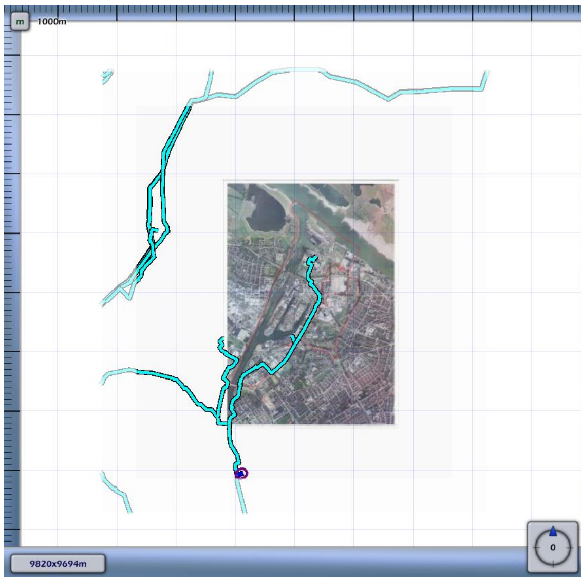
3.11 Figuur 3.11 Plaatsgebonden risico voor N-576-69 van N.V. Nederlandse Gasunie
