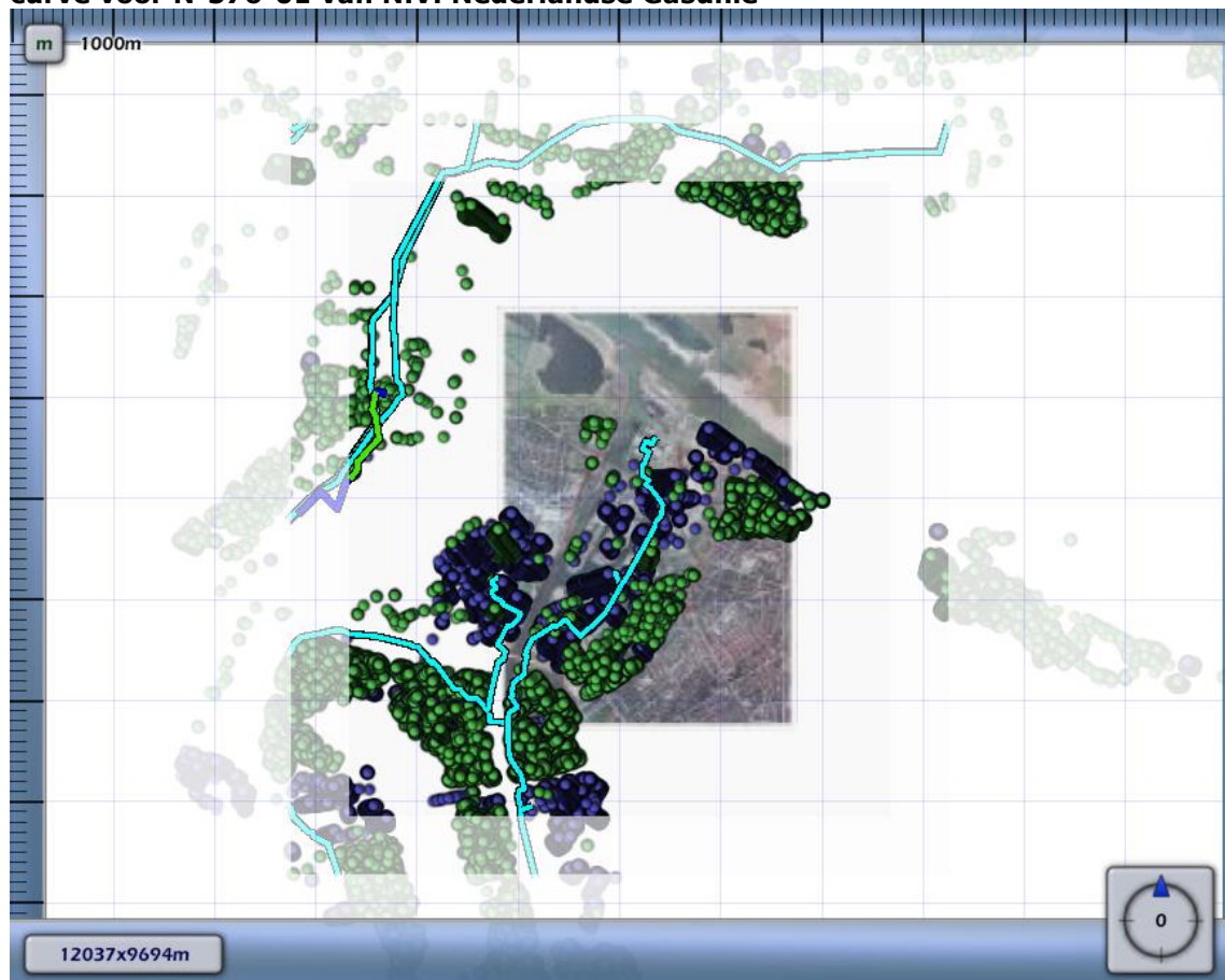
Figuur 4.6 Kilometer leiding behorende bij de maximale overschrijding van de FN-curve voor N-576-01 van N.V. Nederlandse Gasunie
