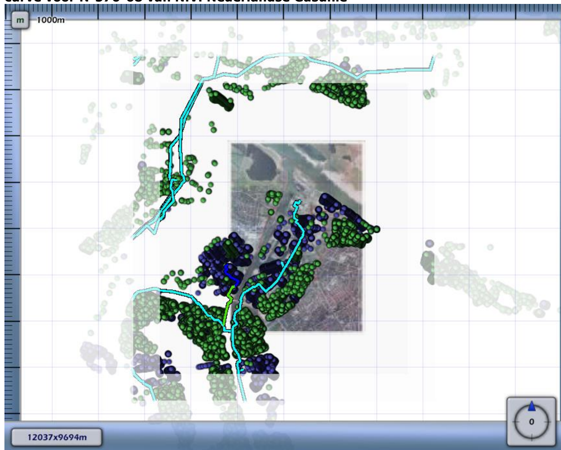
Figuur 4.10 Kilometer leiding behorende bij de maximale overschrijding van de FN-curve voor N-576-68 van N.V. Nederlandse Gasunie
