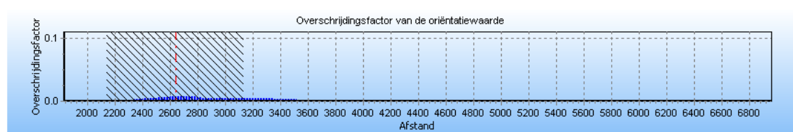
4.9 Figuur 4.9 Groepsrisico screening voor N-576-67 van N.V. Nederlandse Gasunie
